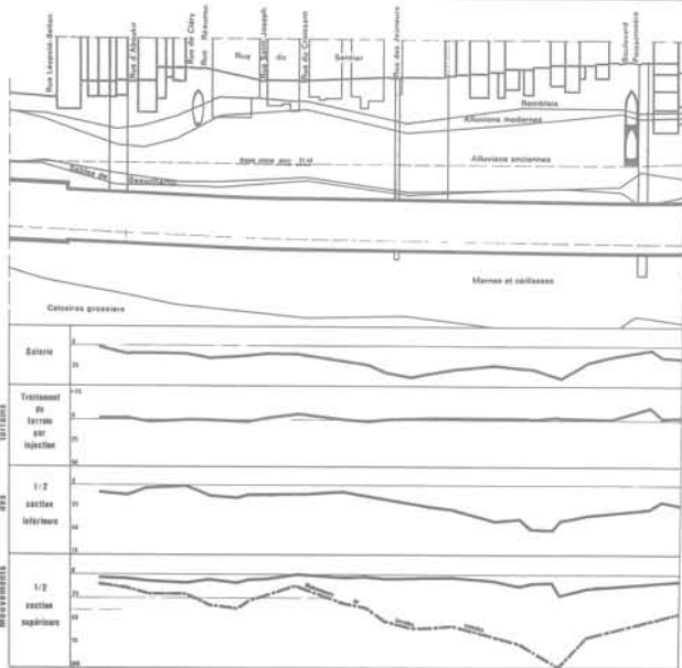
Fig. 11 - Profil en long des mouvements de terrain phase par phase
