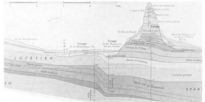
Fig. 4 - Profil en long de la géologie du bassin parisien
