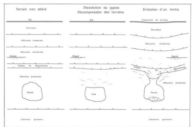
Fig. 6 - Résultat de la dissolution du gypse
