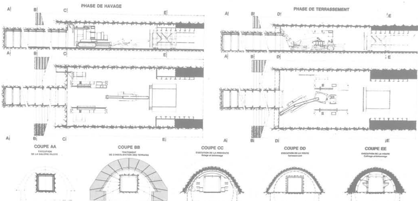
Fig. 7 - Méthode d'exécution de la demi-section supérieure
