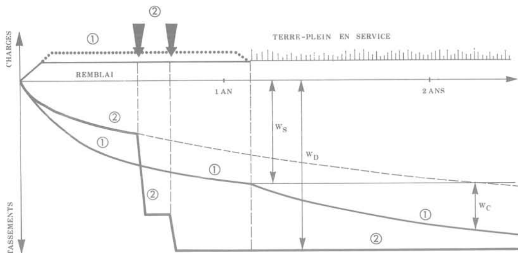
Fig.1 COMPORTEMENT D'UN REMBLAI SUR SOL COMPRESSIBLE.
