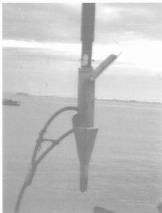
FIG. 2 Système d'ancrage à forte capacité de tenue expérimenté en vraie grandeur en fonds marins coralliens.
