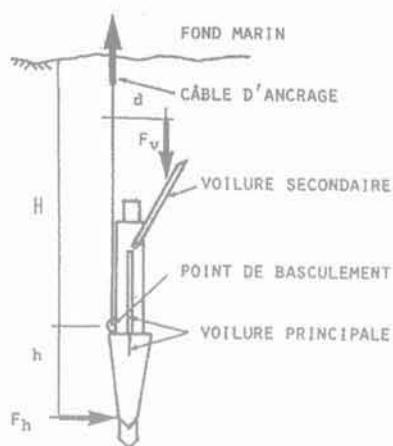
FIG. 1 Description et caractéristiques géométriques du système d'ancrage à forte capacité de tenue testé.
