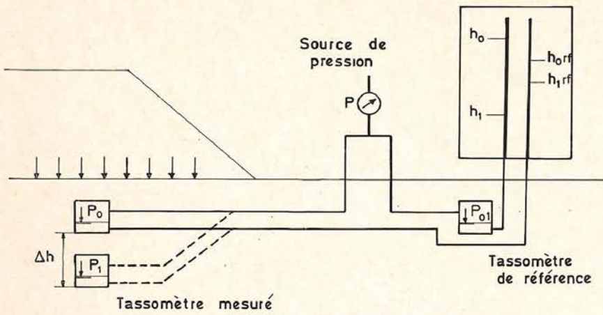
Fig. 3. — Schéma d'installation d'un tassomètre.
