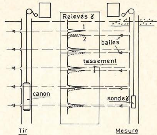
Fig. 4. — Tassomètre à balles radioactives (procédé Syminex, dessin d'après Technical Doc. 201. Syminex-January 1976).
