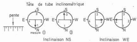
Fig. 10. — Le relevé des faces 1-3 et 4-2 permet de supprimer l'erreur systématique par le calcul.
