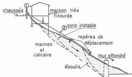
Fig. 24. — Dispositif d'alerte à câble installé sur un talus en Alsace.
