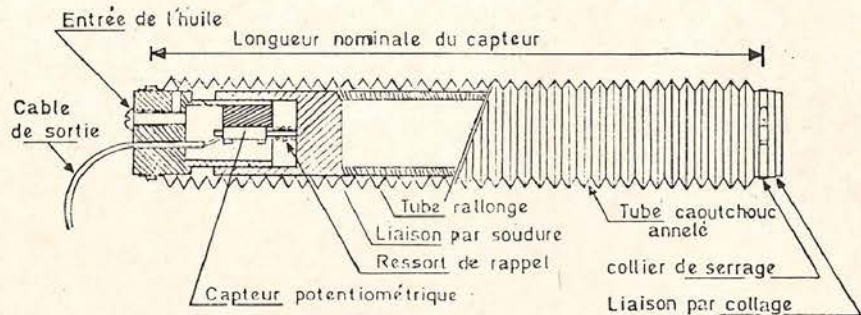
Fig. 6. — Schéma d'un extensomètre.
