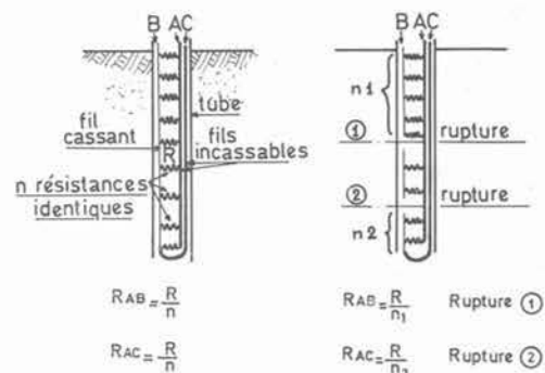
Fig. 19. — Principe du détecteur de profondeur de rupture. Il permet de connaître la profondeur de zones de rupture.
