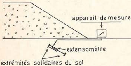
Fig. 5. — Principe d'utilisation de l'extensomètre.
