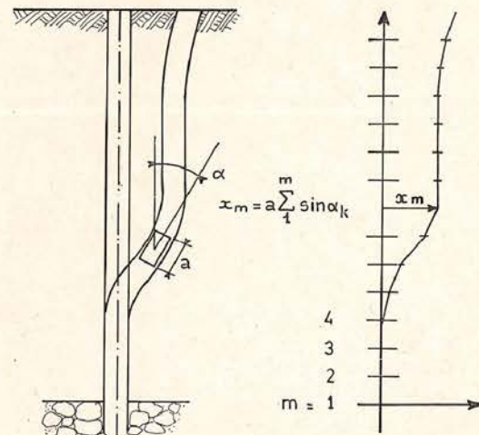
Fig. 7. — Principe de l'inclinomètre.
