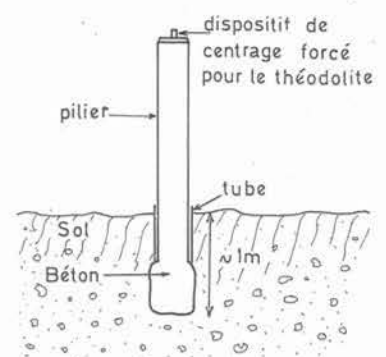
Fig. 15. — Schéma d'un pilier de station insensible aux mouvements superficiels du terrain.
