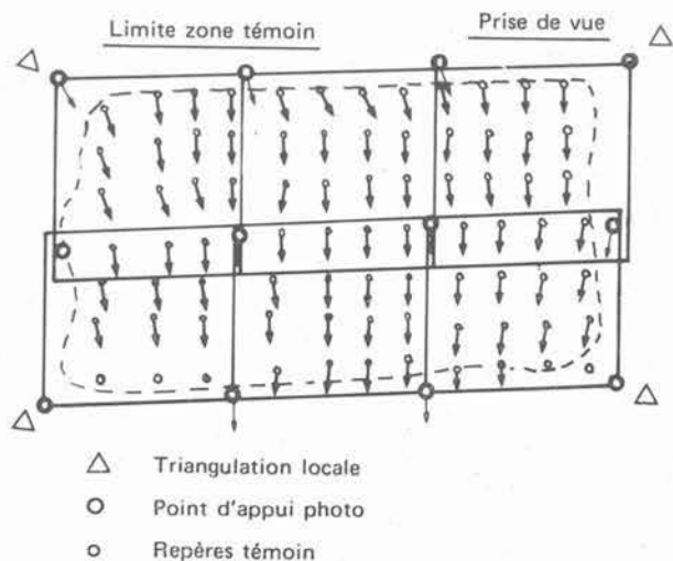
Fig. 17. — Schéma général d'un canevas de prises de vues photogrammétriques.
