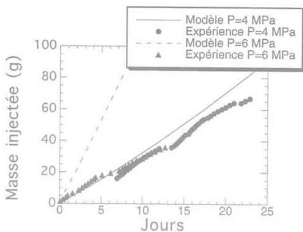
FIG. 9 Masse injectée calculée pour les deux paliers gaz de 4 et 6 MPa en considérant un modèle basé sur le déplacement d'un front de saturation. Calculated injected mass for 4 and 6 MPa pressure steps considering a mobile boundary gas/brine.
