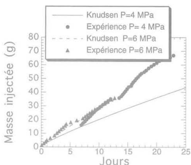
FIG. 8 Masse injectée calculée pour les deux paliers gaz de 4 et 6 MPa en considérant un écoulement Knudsen. Calculated injected mass for 4 and 6 MPa pressure steps considering a Knudsen's flow.
