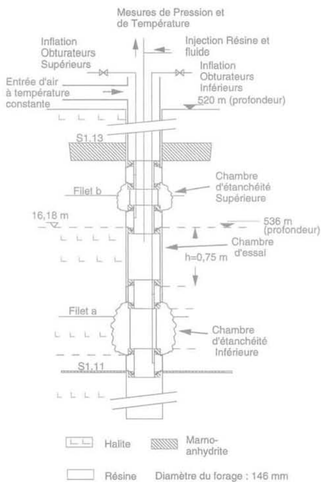
FIG. 3 Équipement du forage d'essai. Borehole equipment.
