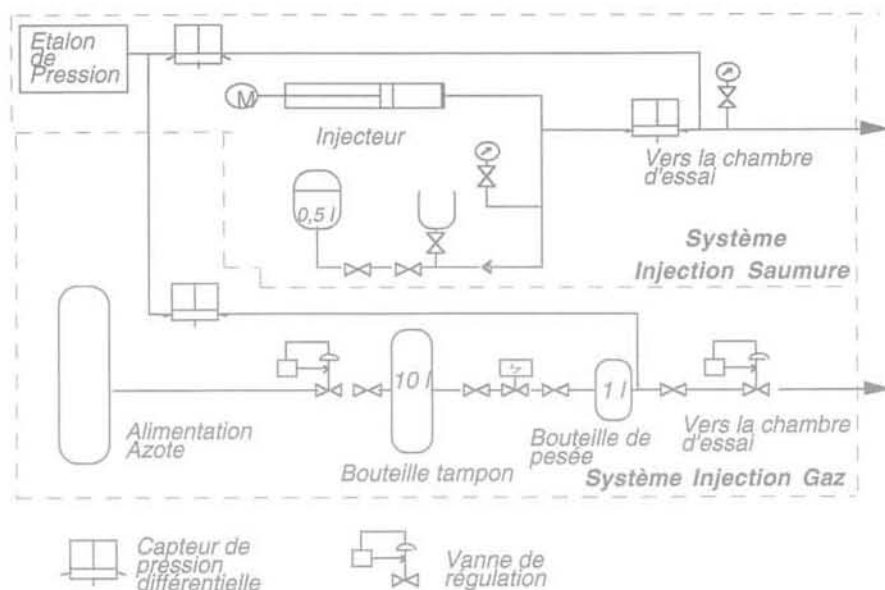
FIG. 2 Systèmes d'injection de fluide (gaz et saumure). Fluid injection systems (gas and brine).
