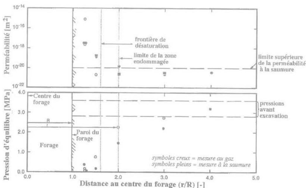
FIG. 1 Évolution de la perméabilité et de la pression de pores dans le sel en fonction de la distance à la paroi du forage (d'après Stormont et al. , 1991 sur le site du Waste Isolation Pilot Plant, États-Unis). Permeability and pore pressure versus distance from borehole wall (Stormont et al. , 1991 on the Waste Isolation Pilot Plant site, USA).
