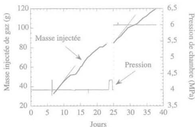
FIG. 6 Masse injectée de gaz au cours de deux paliers de pression, 4 et 6 MPa. Injected gas mass during two pressure steps, 4 and 6 MPa.
