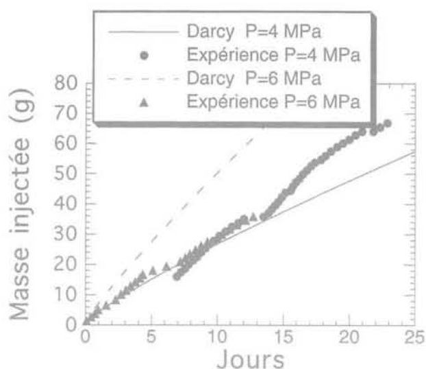
FIG. 7 Masse injectée calculée pour les deux paliers gaz de 4 et 6 MPa en considérant la loi de Darcy. Calculated injected mass for 4 and 6 MPa pressure steps considering a Darcy's law.
