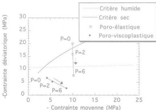
FIG. 5 Position des états de contrainte imposés à la paroi du forage par rapport aux critères d'endommagement du sel. Position of Stress States on the Borehole Wall with respect to the Salt Damage Criteria.
