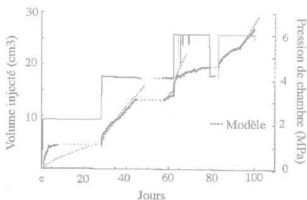
FIG. 4 Comparaison entre les données expérimentales et le modèle tenant compte du régime transitoire pour les valeurs de perméabilité de 2 \cdot 10^{-21} \text{ m}^2 et de pression de pores initiale de 1 MPa. Comparison between experimental data and model. Transient state is taken into account with the values of permeability and pore pressure equal to 2 \cdot 10^{-21} \text{ m}^2 and 1 MPa respectively.
