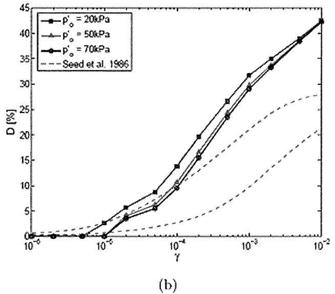
FIG. 5 Comparaison entre la simulation et les courbes de références obtenues par Seed et al. (1986). a) G/G_{\max} - \gamma et b) D - \gamma .
