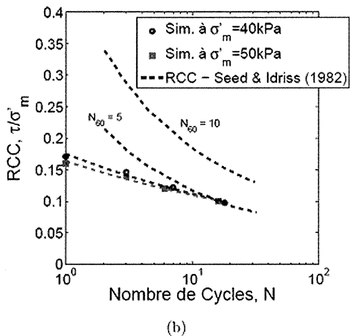
FIG. 6 a) Réponse obtenue lors de la simulation d'un essai cyclique non drainé et b) courbes obtenues pour la résistance au cisaillement cyclique (RCC).
