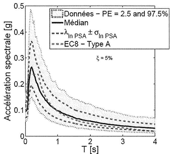
FIG. 4 Spectre de réponse pour les signaux d'entrée.
