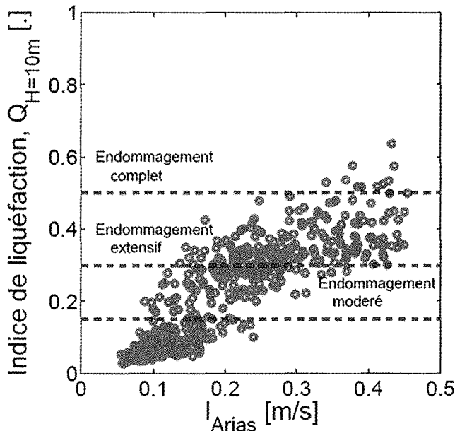
FIG. 10 Diagramme de valeurs obtenues de Q_{H=10} en fonction de I_{Arias} (champ libre).
