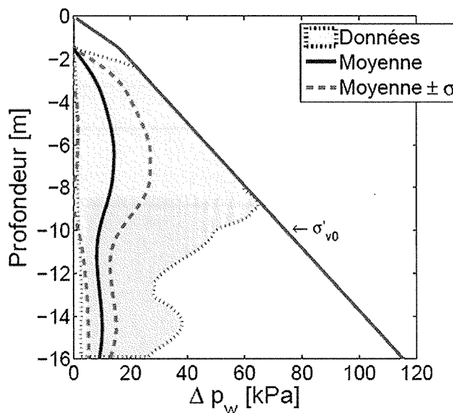
FIG. 7 Increment de la pression interstitielle obtenu dans le profil de sol (champ libre).
