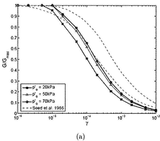
FIG. 5 Comparaison entre la simulation et les courbes de références obtenues par Seed et al. (1986). a) G/G_{\max} - \gamma et b) D - \gamma .
