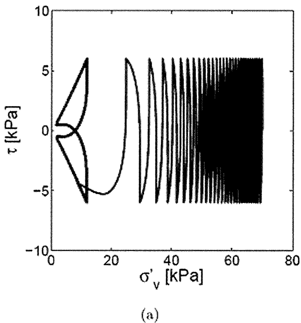
FIG. 6 a) Réponse obtenue lors de la simulation d'un essai cyclique non drainé et b) courbes obtenues pour la résistance au cisaillement cyclique (RCC).
