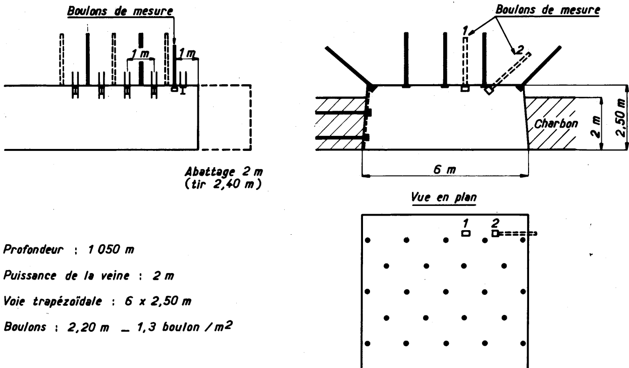
Fig. 4 Wendel – veine 27/28 – Panneau 5 Schéma du boulonnage et implantation des boulons de mesure
