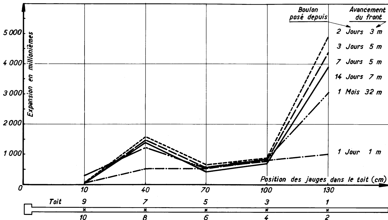
Fig. 6 Wendel – veine 27/28 – Panneau 5 Boulon de mesure n° 1. Allongement en fonction du temps et de l'avancement du front
