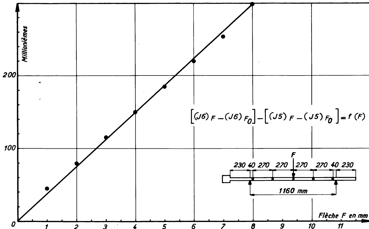
Fig. 3 Etalonnage en flexion
