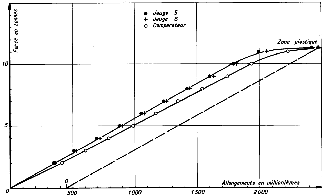
Fig. 2 Etalonnage en traction
