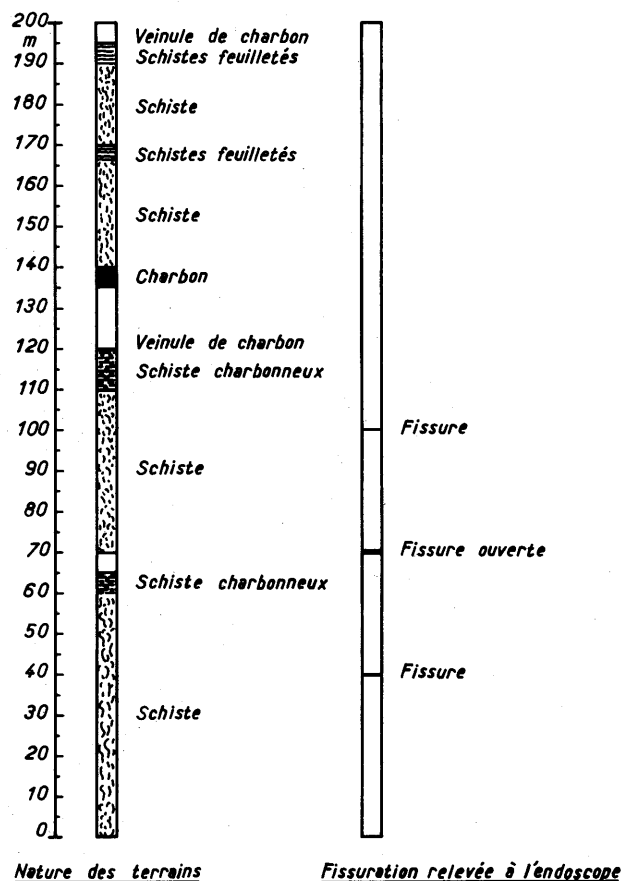
Fig. 5 Wendel – veine 27/28 – Panneau 5 Descenderie de taille. Nature du toit
