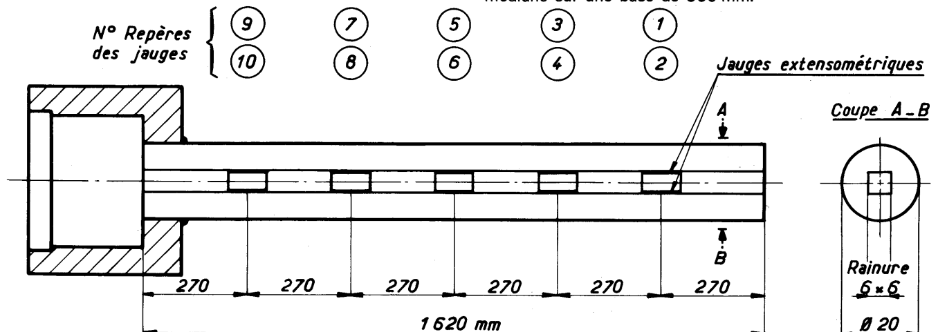
Fig. 1 Boulon de mesure - Coupe longitudinale
