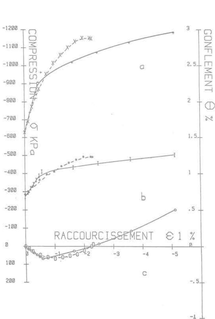
Fig. 13 Comparaison du calcul et de l'expérience pour l'essai de Cornforth, \sigma_3 = 276 KPa
