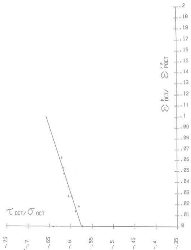
Fig. 1 Etude de la dilatance pendant l'écrouissage pour l'essai A de Al Hussaini
