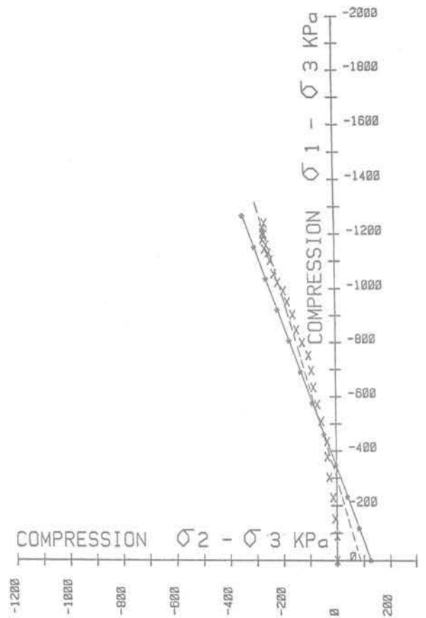
Fig. 10 Etude de la contrainte moyenne calculée et mesurée \sigma_2 pour l'essai C de Al Hussaini
