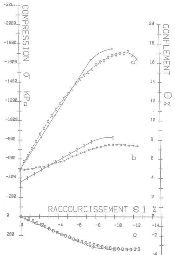
Fig. 16 Comparaison du calcul et de l'expérience pour l'essai C de Al Hussaini, \sigma_3 = 483 KPa
