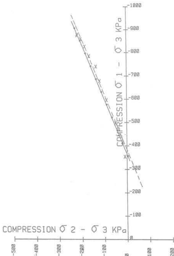
Fig. 7 Etude de la contrainte moyenne calculée et mesurée \sigma_2 pour l'essai de Cornforth
