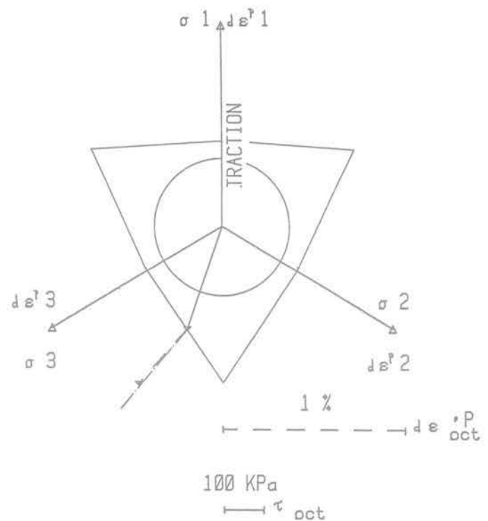
Fig. 5 Etude de la distorsion plastique dans le plan octaédrique pour l'essai CT1 - D2 de Lade
