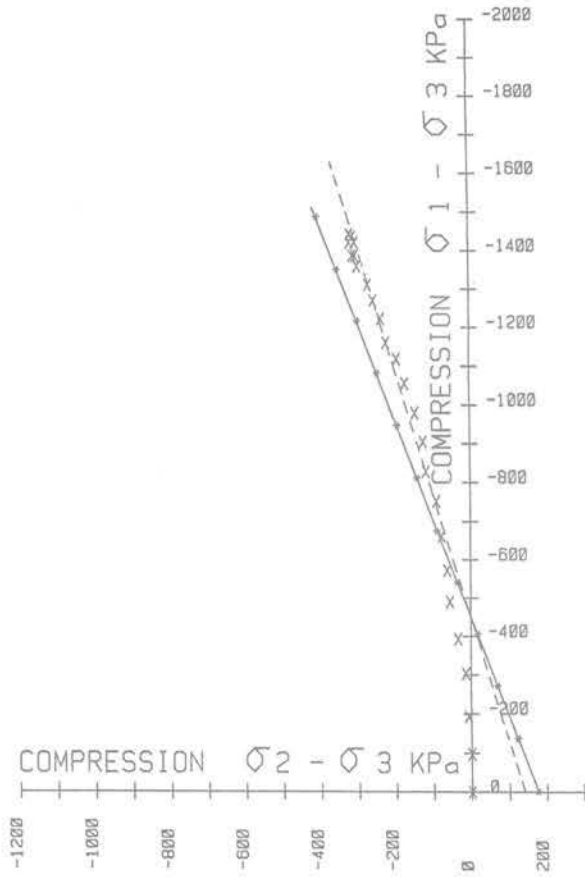
Fig. 9 Etude de la contrainte moyenne calculée et mesurée \sigma_2 pour l'essai B de Al Hussaini
