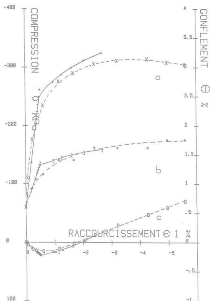
Fig. 18 Comparaison du calcul et de l'expérience pour l'essai CT1 - L2 de Lade, \sigma_3 = 60 \text{ KPa}
