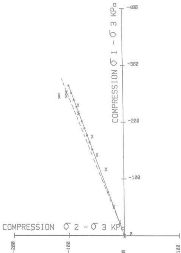
Fig. 11 Etude de la contrainte moyenne calculée et mesurée \sigma_2 pour l'essai CT1 - L2 de Lade
