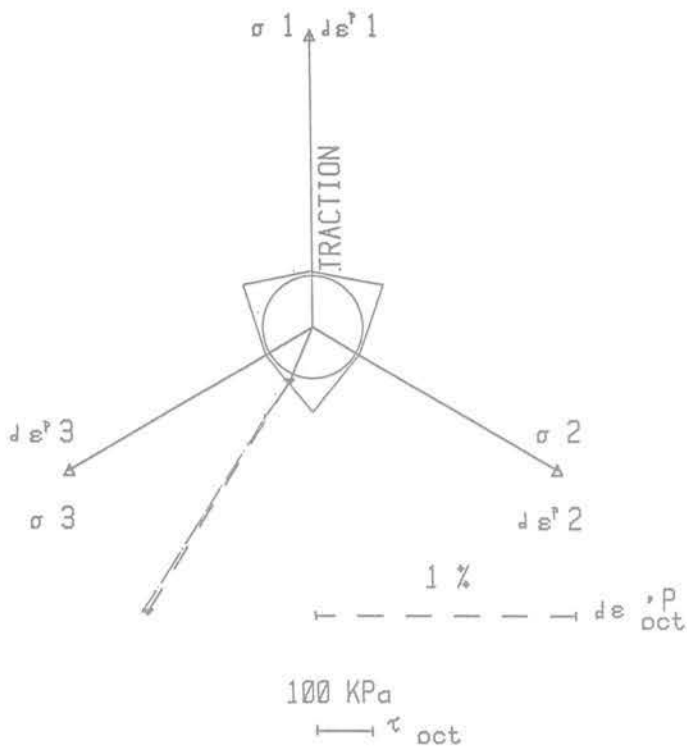
Fig. 4 Etude de la direction plastique dans le plan octaédrique pour l'essai CT1 - L2 de Lade
