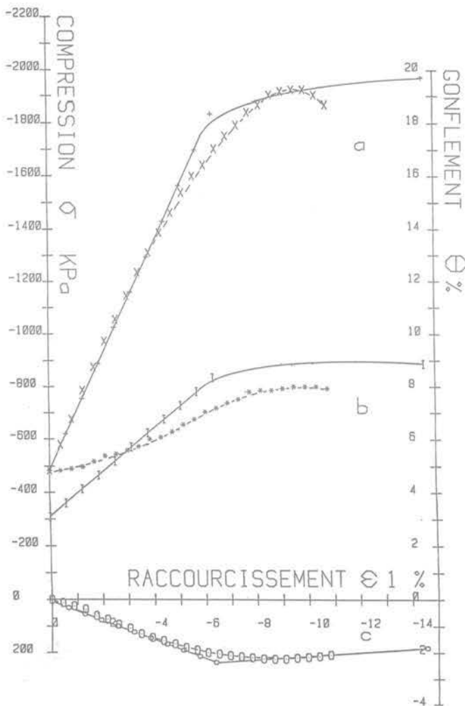
Fig. 15 Comparaison du calcul et de l'expérience pour l'essai B de Al Hussaini, \sigma_3 = 483 KPa
