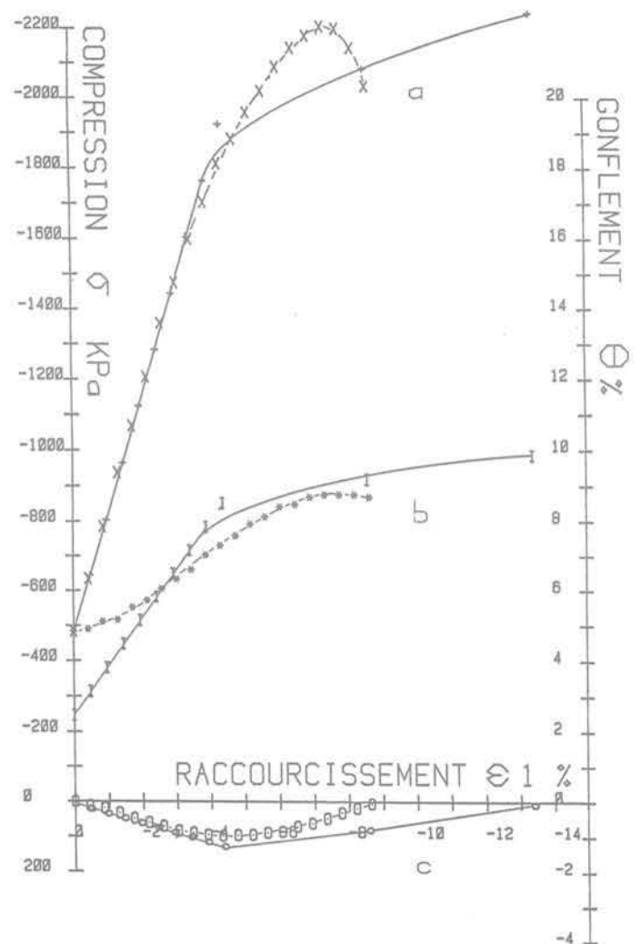
Fig. 14 Comparaison du calcul et de l'expérience pour l'essai A de Al Hussaini, \sigma_3 = 483 KPa
