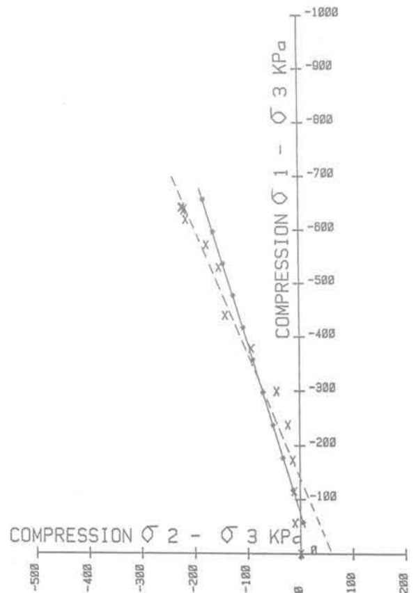
Fig. 12 Etude de la contrainte moyenne calculée et mesurée \sigma_2 pour l'essai CT1 - D2 de Lade
