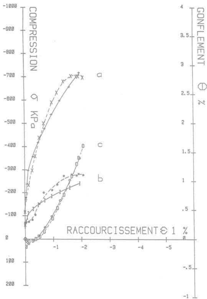
Fig. 17 Comparaison du calcul et de l'expérience pour l'essai CT1 - D2 de Lade, \sigma_3 = 60 \text{ KPa}
