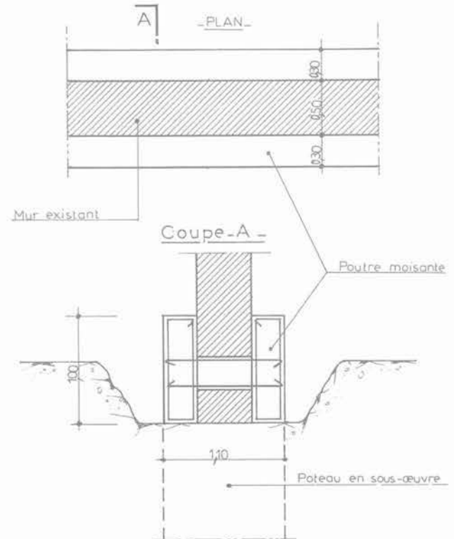
Fig. 18. — Paris 8 e . Rue Paul-Baudry. Détails poutre moisante.
