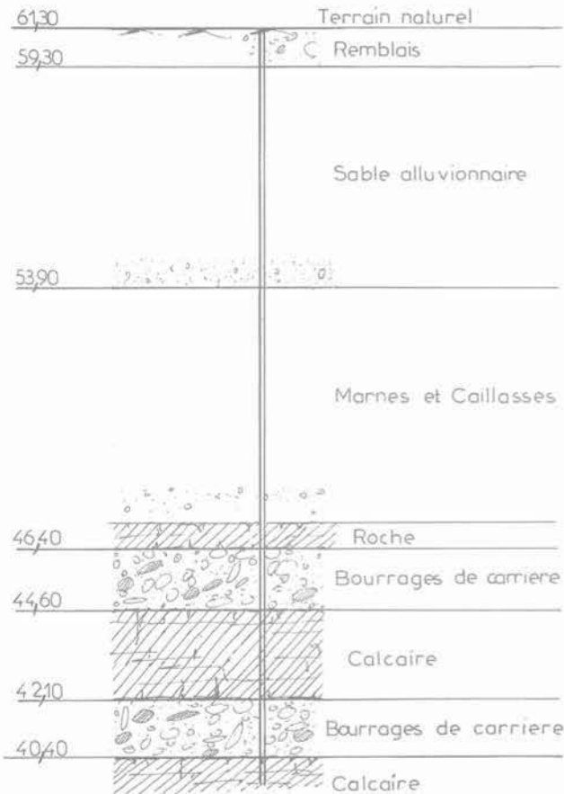
Fig. 21. — Ivry-sur-Seine. Coupe géologique.
