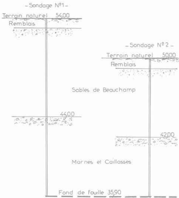
Fig. 9. — Paris 8 e . Rues Galilée-Vernet. Coupes géologiques.
