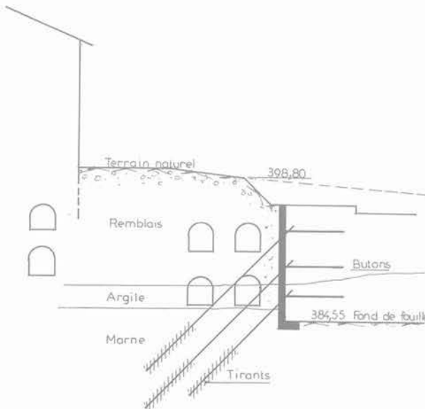
Fig. 13. — Clermont-Ferrand. Avenue Georges-Clemenceau, coupe amont.
