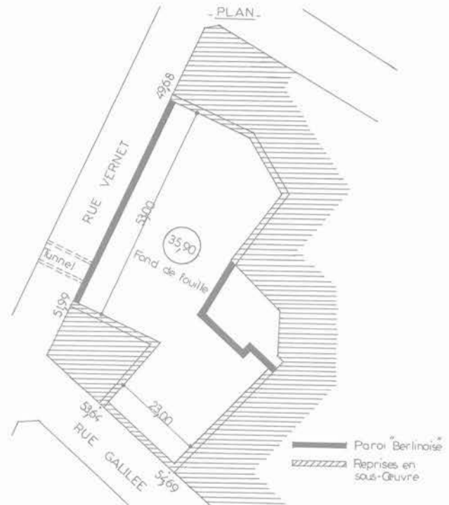
Fig. 10. — Paris 8 e . Rues Galilée-Vernet.
