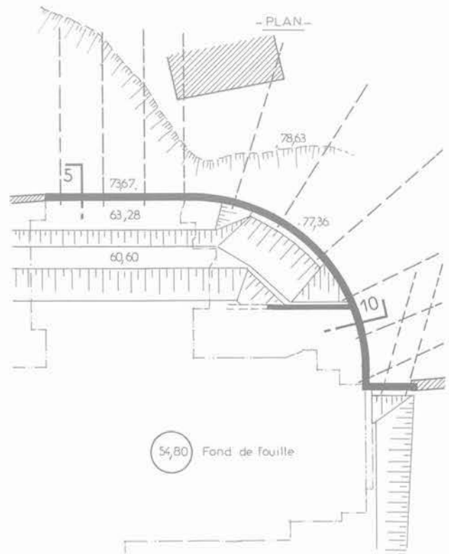
Fig. 2. — Sèvres - 170, Grande Rue. Bâtiment B.
