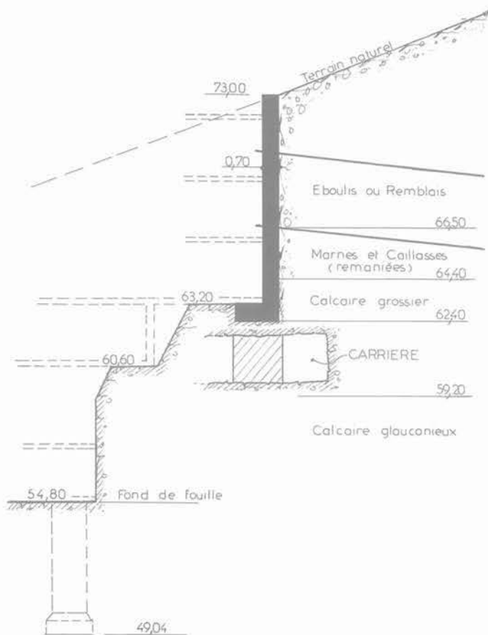
Fig. 3. — Sèvres - 170, Grande Rue. Bâtiment B, coupe 5.
