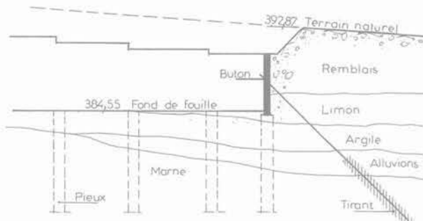
Fig. 14. — Clermont-Ferrand. Avenue Georges-Clemenceau, coupe aval.
