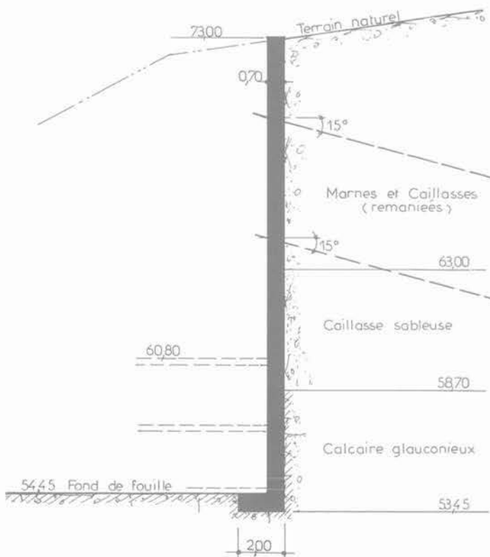
Fig. 1. — Sèvres - 170, Grande Rue. Bâtiment B, coupe 10.
