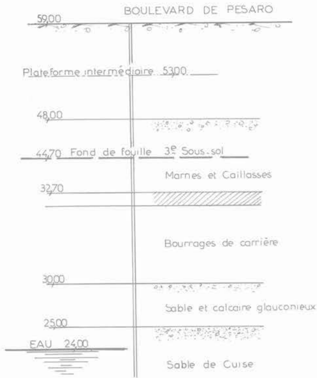
Fig. 5. — Nanterre. Bâtiment MB7, coupe géologique.
