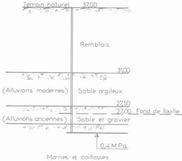
Fig. 16. — Paris 8 e . Rue Paul-Baudry, coupe géologique.
