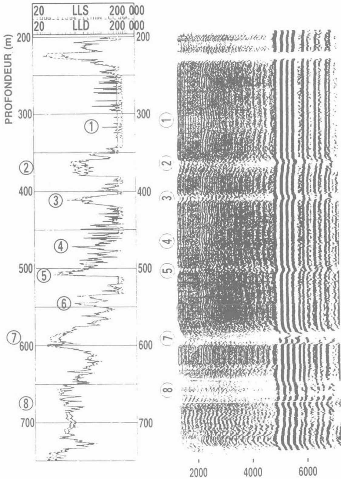
Fig. 7. — Section iso-offset comparée à des diagraphies de résistivité dans le granit (puits A). Fig. 7. — Iso-offset section versus resistivity logs in granite (well A).
