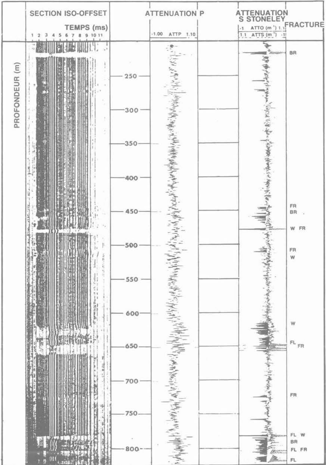
Fig. 8. — Détection de fractures avec EVA dans du granit (puits B).
