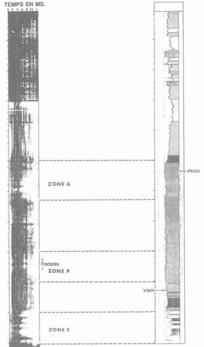
Fig. 11. — Section iso-offset et colonne lithologique tirée d'EVA pour Gaviota 5.
