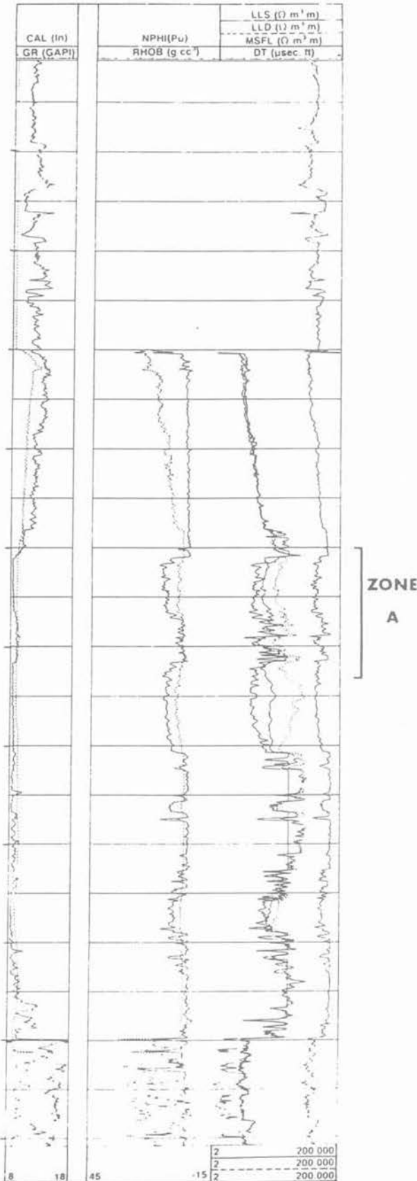
Fig. 10. — Diagraphies conventionnelles pour Gaviota 5. Fig. 10. — Conventional logs for Gaviota 5.
