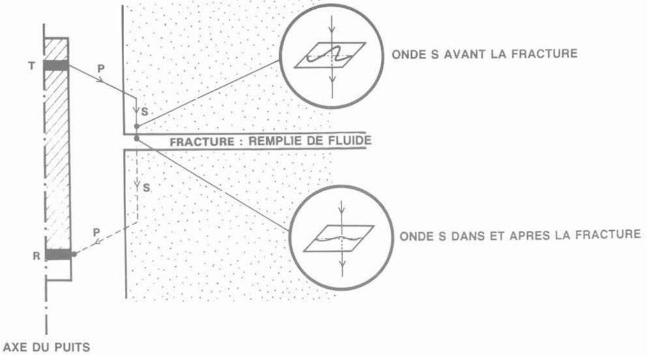
Fig. 9. — Modèle physique simple pour la propagation d'une onde S à travers une fracture. Fig. 9. — Simple physical model for the propagation of an S wave through a fracture.
