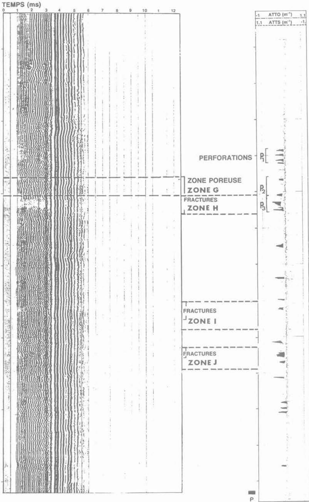
Fig. 15. — Résultats complets pour Gaviota 7. Fig. 15. — Complete results for Gaviota 7.
