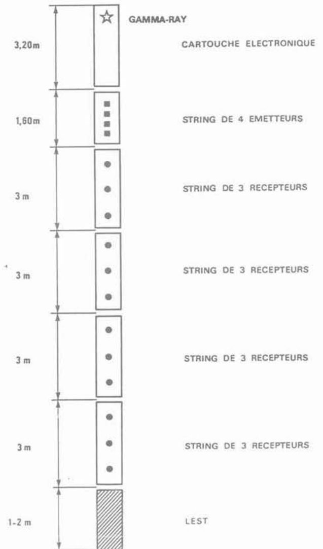
Fig. 1. — Diagramme schématique de l'outil. Fig. 1. — Tool schematic Diagram.
