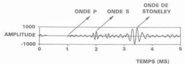
Fig. 2. — Exemple d'un trajet enregistré. Les trois types d'ondes (P, S, Stoneley) sont visibles.
