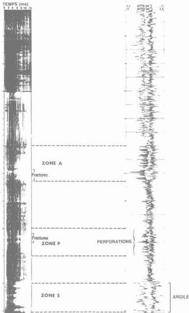
Fig. 12. — Section iso-offset et diagraphie de fracturation pour Gaviota 5, avec indication des zones perforées. Fig. 12. — Iso-offset section and fracturation log for Gaviota 5 with indication of perforated zone.
