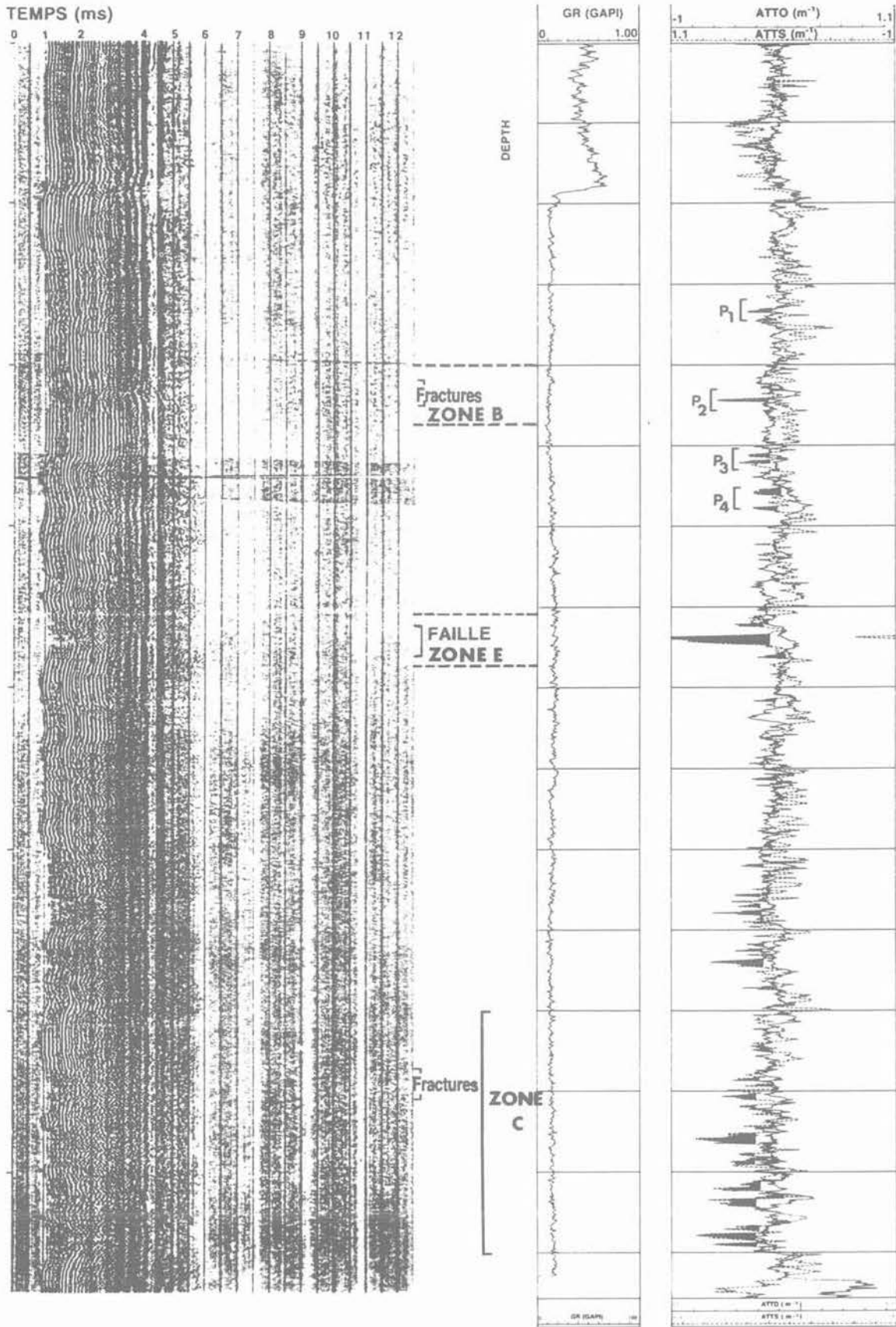
Fig. 14. — Diagraphie de fracturation et section-offset pour Gaviota 6, avec indication des zones perforées.
