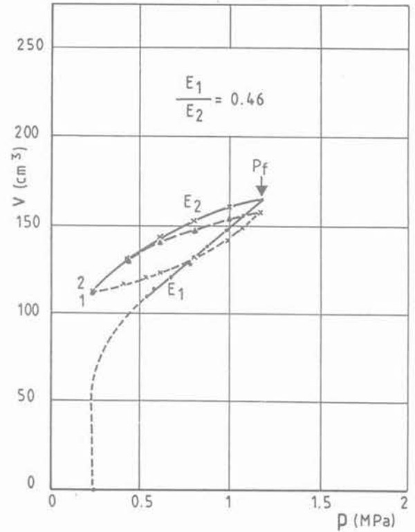
Fig. 11. — Pressiomètre cyclique sous la fondation - z = 20 cm Fig. 11. — Cyclic pressuremeter tests under the foundation, z = 20 m
