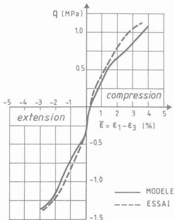
Fig. 4a. — Gault inférieur - Essais triaxiaux non drainés - Calage du modèle.
