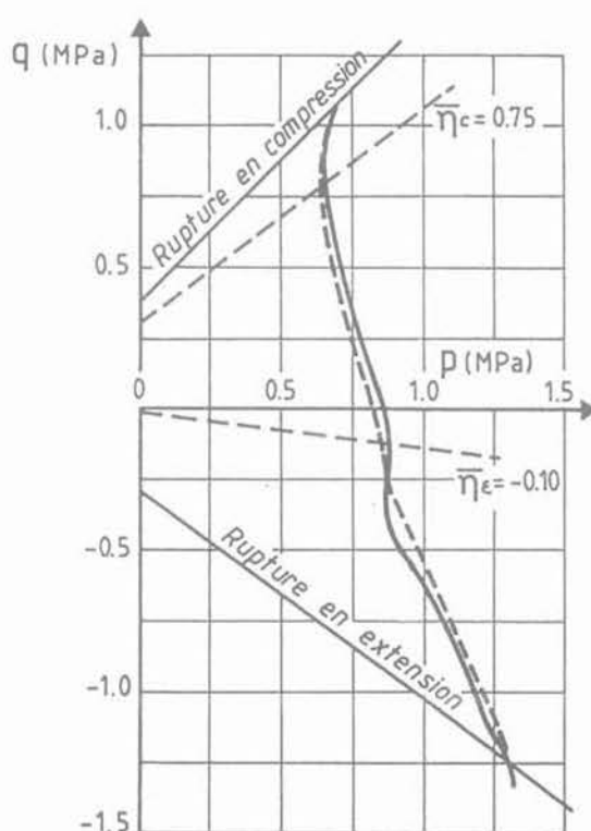
Fig. 4b. — Gault inférieur - Essais triaxiaux non drainés - Calage du modèle.
