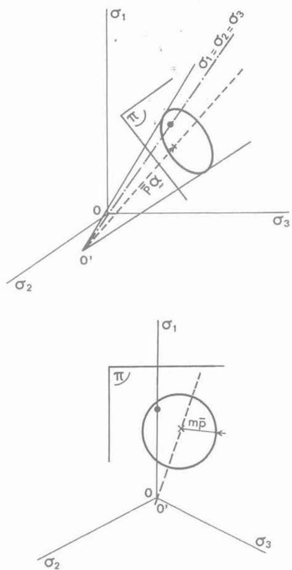
Fig. 2. — Surface de charge dans l'espace des contraintes effectives principales. Fig. 2. — Yield surface in the principle effective stress space.
