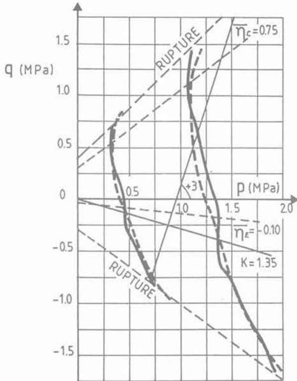
Fig. 6b. — Gault inférieur. Essais triaxiaux non drainés. Fig. 6b. — Lower Gault - Undrained triaxial tests.
