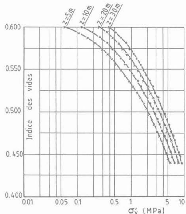
Fig. 9. — Œdomètres sous la fondation - Calcul numérique. Fig. 9. — Compressibility tests under the foundation - numerical calculation.
