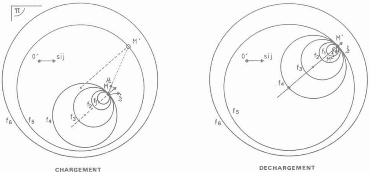
Fig. 3. — Ecrouissage cinématique du modèle à surfaces multiples. Fig. 3. — Kinematic hardening of the multiple yield surface model.
