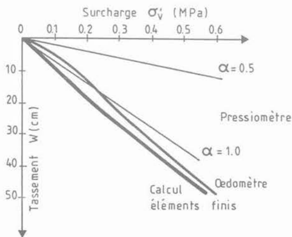
Fig. 13. — Comparaison des tassements calculés par E.F. et prévus.
