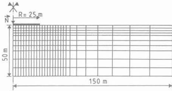
Fig. 12. — Maillage éléments finis. Fig. 12. — Finite element mesh.
