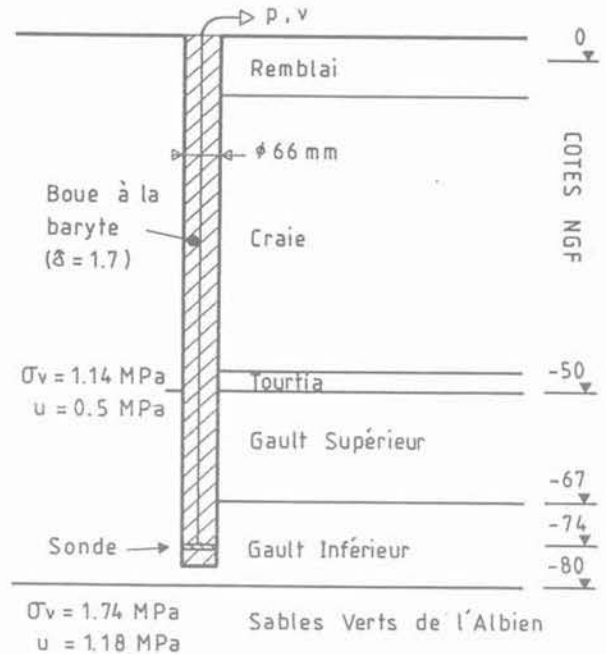
Fig. 1. — Site de Penly - Stratigraphie.
