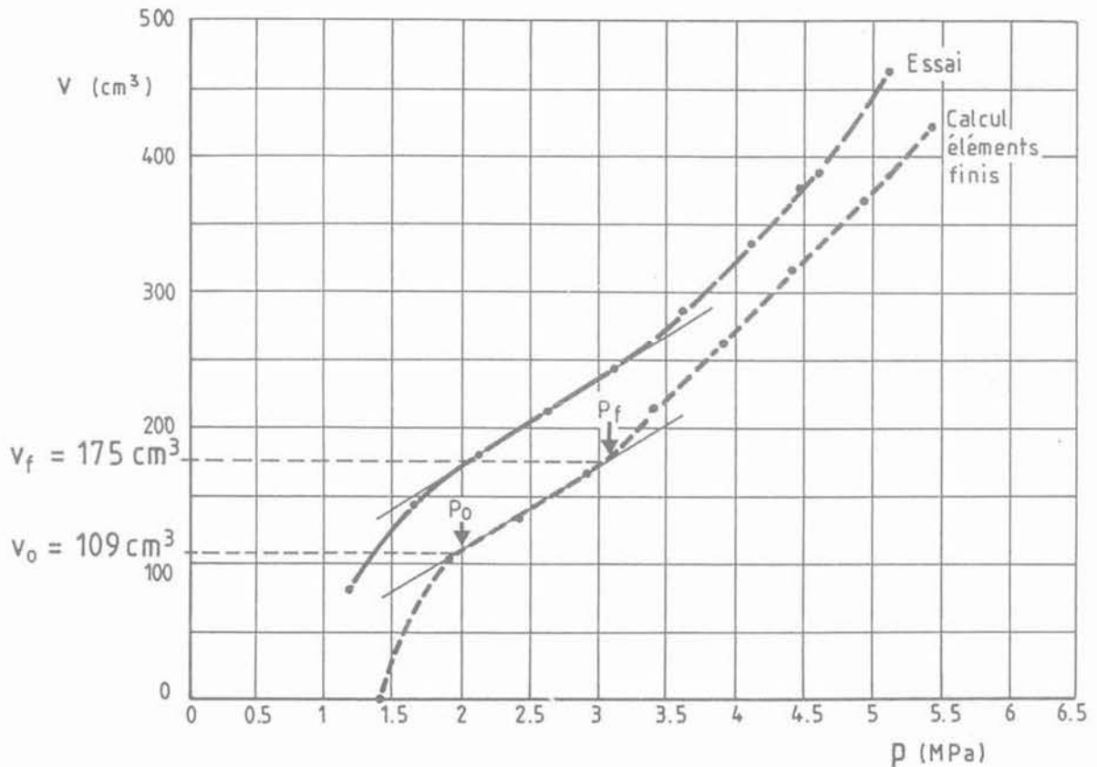
Fig. 8. — Essai pressiométrique réalisé à Penly - Cote : - 74 NGF.
