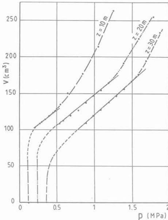
Fig. 10. — Pressiomètres sous la fondation - Calcul numérique. Fig. 10. — Pressuremeter tests under the foundation - numerical calculation.
