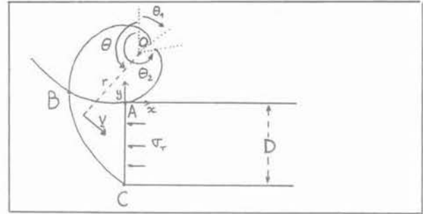
Fig. 6. — Allure du mécanisme à deux spirales. Fig. 6. — Geometrical aspect of the two spirals mechanism.
