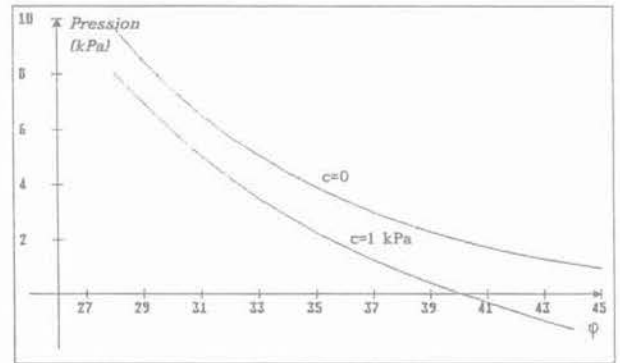
Fig. 4. — Pression limite en fonction de l'angle de frottement. Effet de la cohésion à densité fixée (16 kN/m 3 ) et pour un diamètre de 5 m. Fig. 4. — Limit pressure versus friction angle: influence of cohesion for a given density and for a 5 m diameter tunnel.
