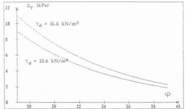
Fig. 3. — Estimation de la pression limite en fonction de l'angle de frottement, pour une cohésion nulle. Effet de la densité pour un diamètre de 5 m. Fig. 3. — Limit pressure evaluation versus friction angle for a non cohesive material; density influence for a 5 m diameter tunnel.
