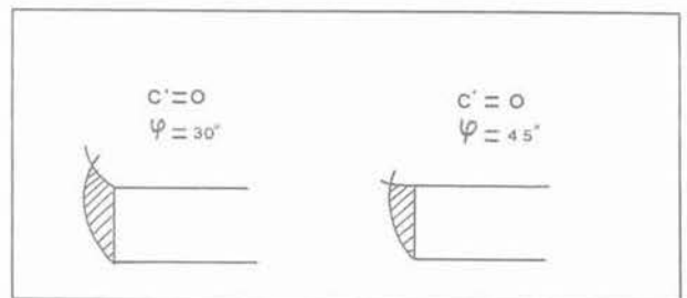
Fig. 8. — Mécanismes optimaux pour différents angles de frottement. Fig. 8. — Optimal mechanisms for various friction angles.
