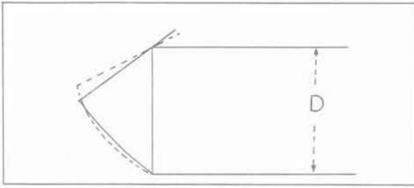
Fig. 5. — Mécanismes pour deux angles de frottement différents: \varphi = 30^\circ (pointillé) et \varphi = 40^\circ (trait plein). Fig. 5. — Two mechanisms corresponding to different friction angles: \varphi = 30^\circ (dotted line), \varphi = 40^\circ (continuous line).
