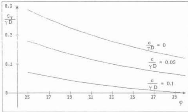
Fig. 9. — Influence de la cohésion et de l'angle de frottement sur la pression limite de soutien.
