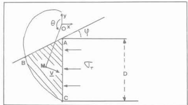
Fig. 2. — Configuration géométrique du mécanisme à une spirale. Fig. 2. — Geometrical aspect of the one spiral mechanism.
