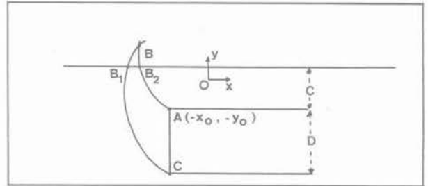
Fig. 11. — Configuration géométrique dans le cas où l'influence de la surface est prise en compte.
