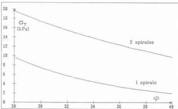
Fig. 10. — Comparaison des valeurs données par les deux mécanismes pour c = 0 , \gamma_d = 16 \text{ kN/m}^3 et D = 5 \text{ m} .
