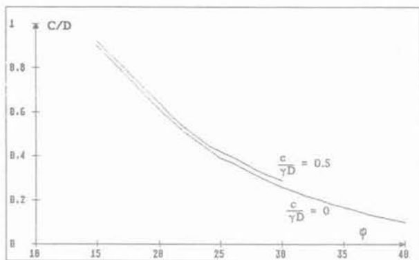
Fig. 12. — Variations de la profondeur critique pour différents angles de frottement et différentes valeurs de la cohésion réduite.
