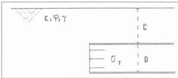
Fig. 1. — Schéma de la cavité. Fig. 1. — Scheme of the cavity.
