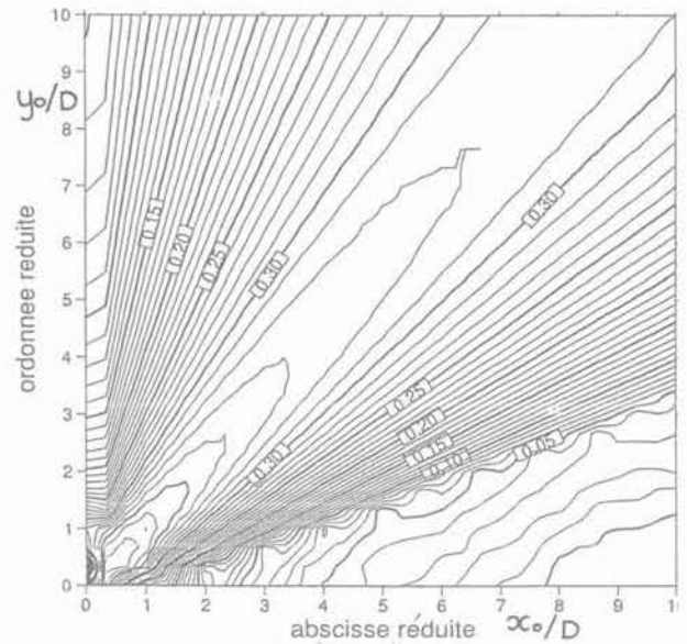
Fig. 7. — Isovaleurs de la pression limite lorsque les coordonnées du centre de spirales varient. Cas d'une cohésion nulle et d'un angle de frottement de 20°. Fig. 7. — Limit pressure values as a function of the location of the spirals origin ( c = 0, \varphi = 20^\circ ).
