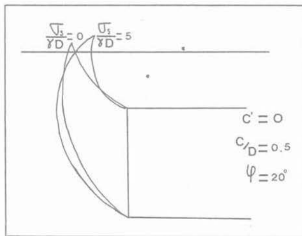
Fig. 14. — Mécanismes avec et sans surcharge ( c = 0, \varphi = 20^\circ ).
