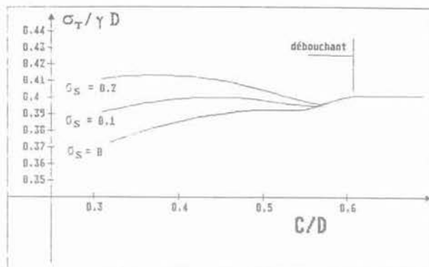
Fig. 13. — Pression limite de soutien avec et sans surcharge ( c = 0, \varphi = 20^\circ ).
