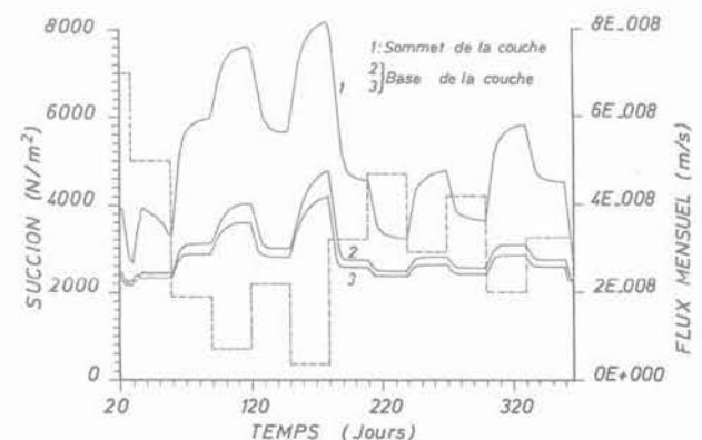
Fig. 8. — Evolution de la succion dans la terre végétale. Fig. 8. — Evolution of suction in loam.
