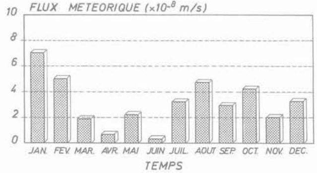
Fig. 6. — Flux moyen mensuel de l'année 1988. (Valeurs obtenues d'après les relevés pluviométriques de Saint-Sauveur-le-Vicomte.)
