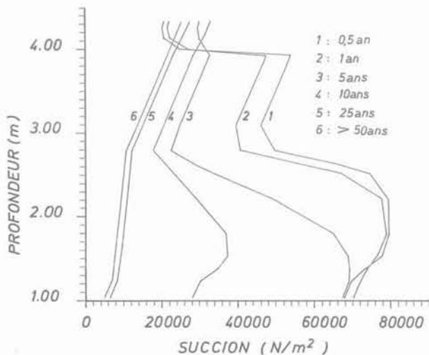
Fig. 10. — Profils d'équilibre de succion (verticale centrale).
