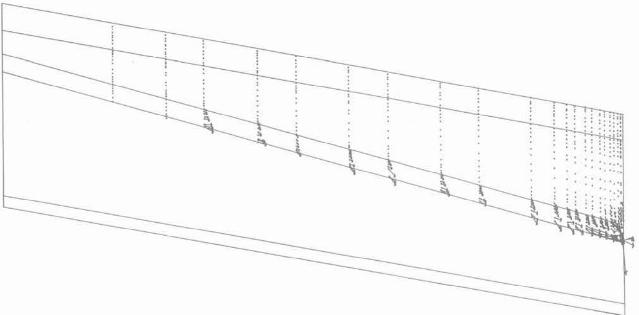
Fig. 13. — Représentation des flux hydrauliques dans le domaine. Simulation avec une condition de succion à la sortie des drains sableux. Flux = Flux mensuel moyen de l'année 1988.
