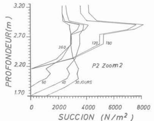
Fig. 7. — Profils de succion pour 3, 5, 10, 15, 30, 40, 60, 120, 180 et 360 jours. Flux = Flux mensuel moyen de l'année 1988.
