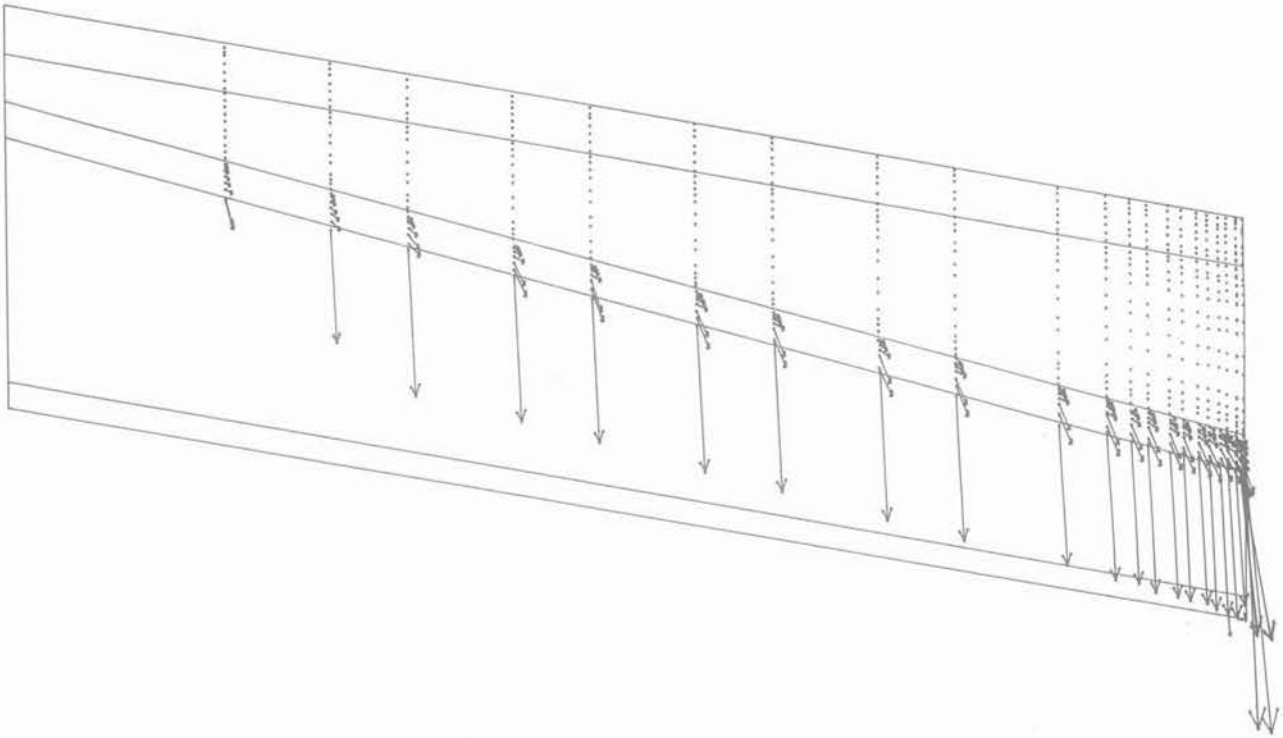
Fig. 11. — Représentation des flux hydrauliques dans le domaine. Simulation avec une condition de surface de suintement à la sortie des drains sableux. Flux = 10^{-8} m/s sur 4 ans.
