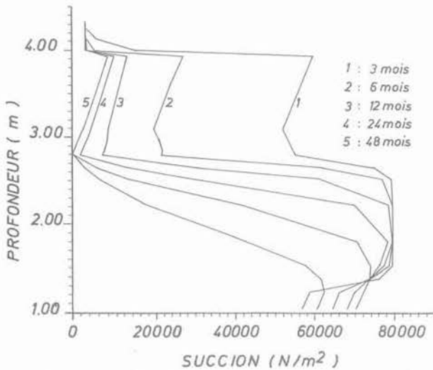
Fig. 9. — Profils d'infiltration sur la verticale centrale pour un flux de 10^{-8} m/s.
