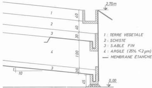
Fig. 1. — Schéma du dispositif.
