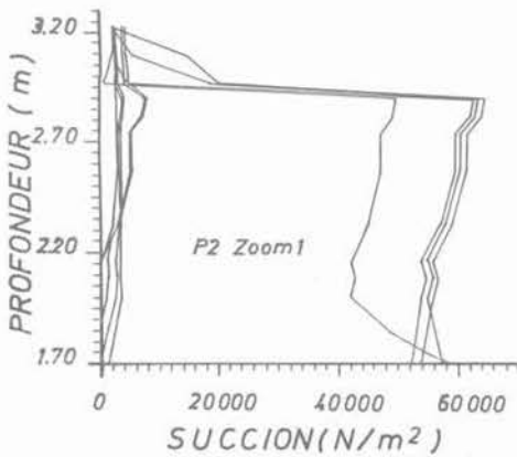
Fig. 7. — Profils de succion pour 3, 5, 10, 15, 30, 40, 60, 120, 180 et 360 jours. Flux = Flux mensuel moyen de l'année 1988.
