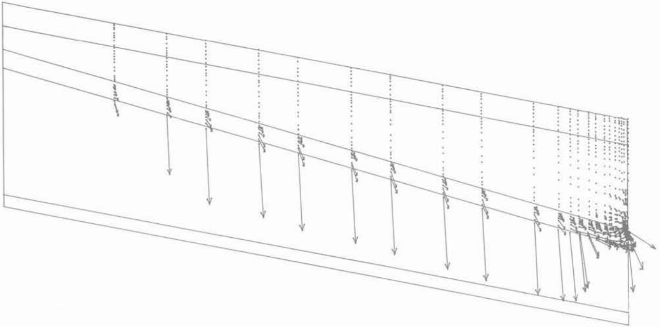
Fig. 12. — Représentation des flux hydrauliques dans le domaine. Simulation avec une condition de succion à la sortie des drains sableux. Flux = 10^{-8} m/s sur 4 ans.
