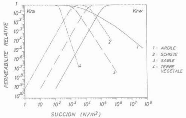
Fig. 3. — Courbes perméabilité relative - succion. Fig. 3. — Curves relative permeability - suction.
