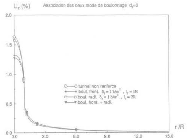
FIG.11-b Convergence axiale pour l'association des deux modes de boulonnage : d_0 = 0 . Axial convergence when associating radial and facing bolts : d_0 = 0 .
