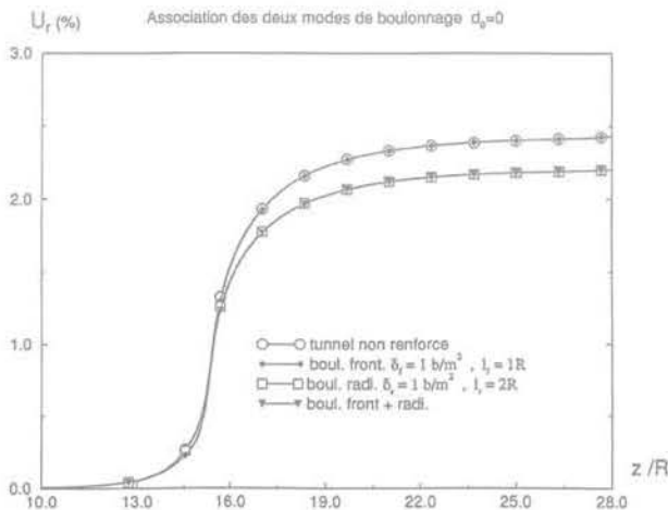
FIG.11-a Convergence radiale pour l'association des deux modes de boulonnage : d_0 = 0 . Radial convergence when associating radial and facing bolts : d_0 = 0 .
