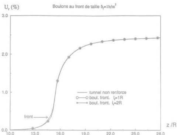
FIG. 8 Convergence le long de l'axe du tunnel, pour deux valeurs de l_r . Convergence profile along the tunnel axis for two values of l_r .
