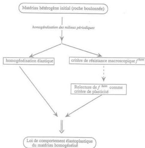
FIG. 3 Démarche suivie pour la formulation du comportement homogénéisé. Procedure to formulate the constitutive law of the homogenized material.
