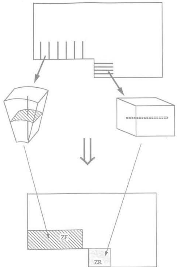
FIG. 2 Volumes représentatifs et problème homogénéisé. Representative elementary volumes and homogenized problem.
