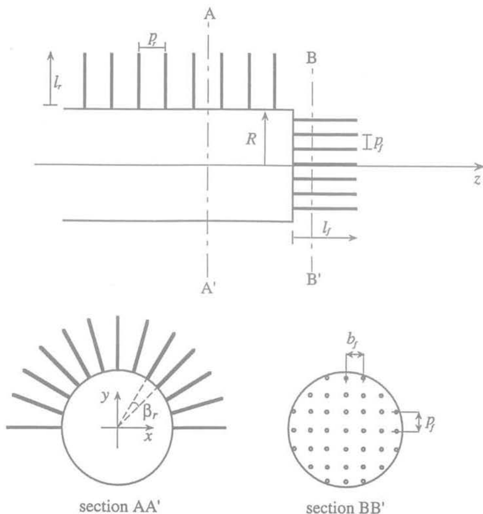
FIG.1 Caractéristiques géométriques du problème. Geometrical characteristics of the problem.
