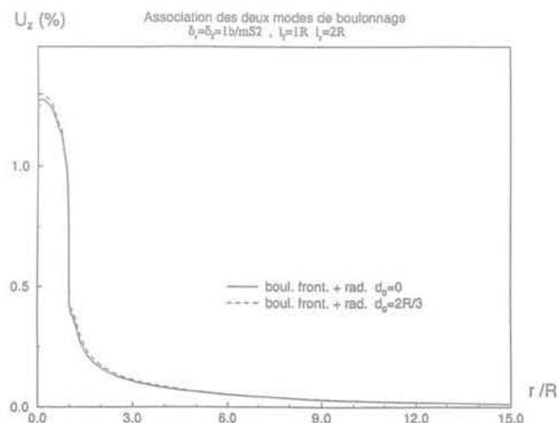
FIG.12: Convergences radiale (a) et axiale (b) pour l'association des deux modes de boulonnage : d_0 = 2R/3 . Radial (a) and axial (b) convergence when associating radial and facing bolts : d_0 = 2R/3 .
