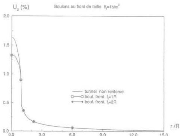
FIG. 9 Convergence axiale en fonction de r . Axial convergence along the r -axis.
