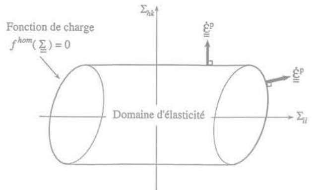
FIG.5 Domaine d'élasticité du matériau homogénéisé et règle d'écoulement. Elasticity domain for the homogenized material and associated flow rule.
