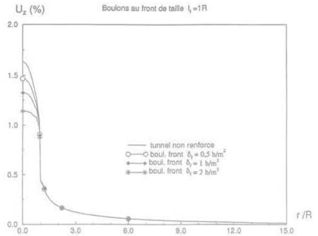
FIG.10 Influence de la densité de boulonnage frontal sur la convergence axiale. Influence of the facing bolt density on the axial convergence.
