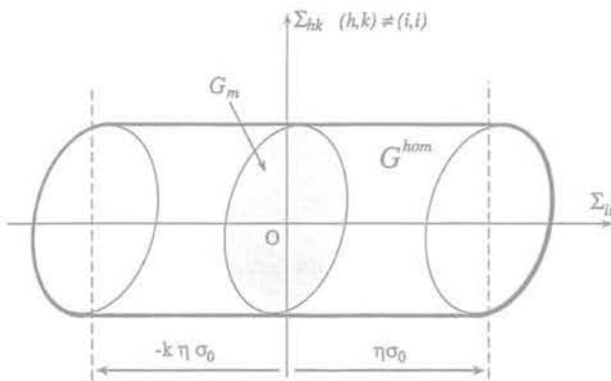
FIG.4 Interprétation géométrique du domaine G^{hom} . Geometrical interpretation of the macroscopic strength domain.
