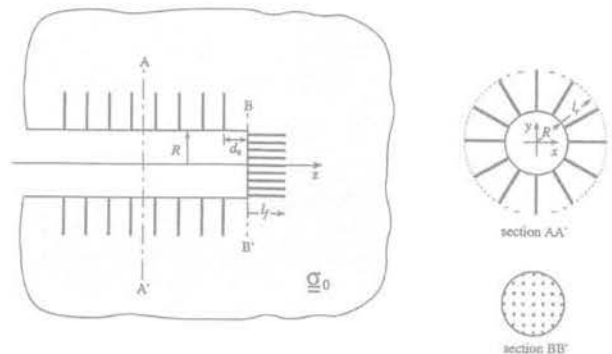
FIG. 6 Tunnel boulonné creusé à grande profondeur dans un milieu isotrope. Bolt supported tunnel excavated at great depth in an isotropic rockmass.
