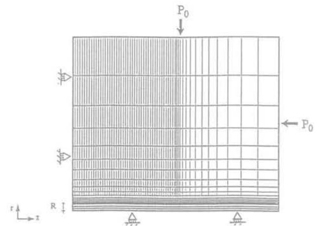
FIG.7 Maillage par éléments finis utilisé. Finite element mesh used.
