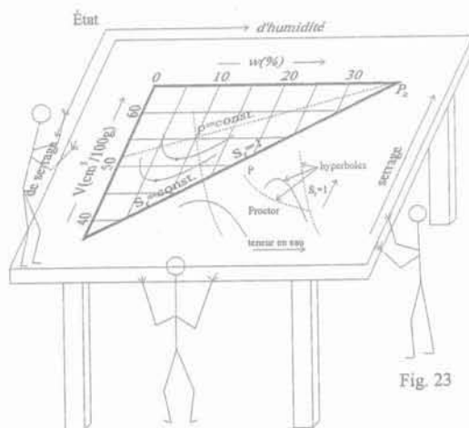
FIG. 23 Schémas concernant les empreintes (a) et les diagrammes d'état (b). Schemas concerning prints (a) and state diagrams (b).
