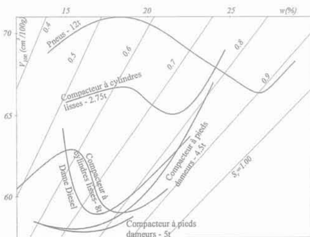
FIG. 18 Diagrammes avec les courbes de compactage d'une argile très plastique. Diagrams with compaction curves of a very plastic clay.
