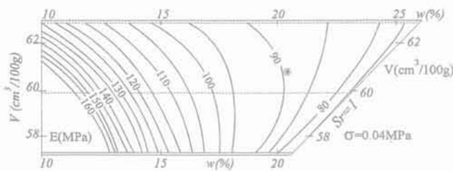
FIG. 22 Diagrammes avec courbes d'égal module dynamique E_d (a) et G_d (b). Diagrams with equal dynamic modulus curves E_d (a) and G_d (b).
