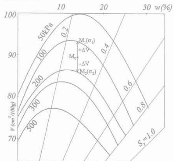
FIG. 10 Diagramme avec les courbes d'équilibre d'état pour différentes pressions normales pendant le cisaillement. Diagram with equilibrium state during direct shear for different normal pressures.
