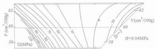
FIG. 22 Diagrammes avec courbes d'égal module dynamique E_d (a) et G_d (b). Diagrams with equal dynamic modulus curves E_d (a) and G_d (b).
