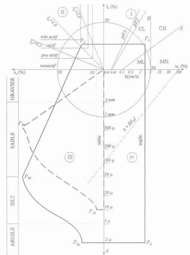
FIG. 1 Les empreintes « A » d'un sable et d'une argile. « A » Prints of a sand and a clay.
