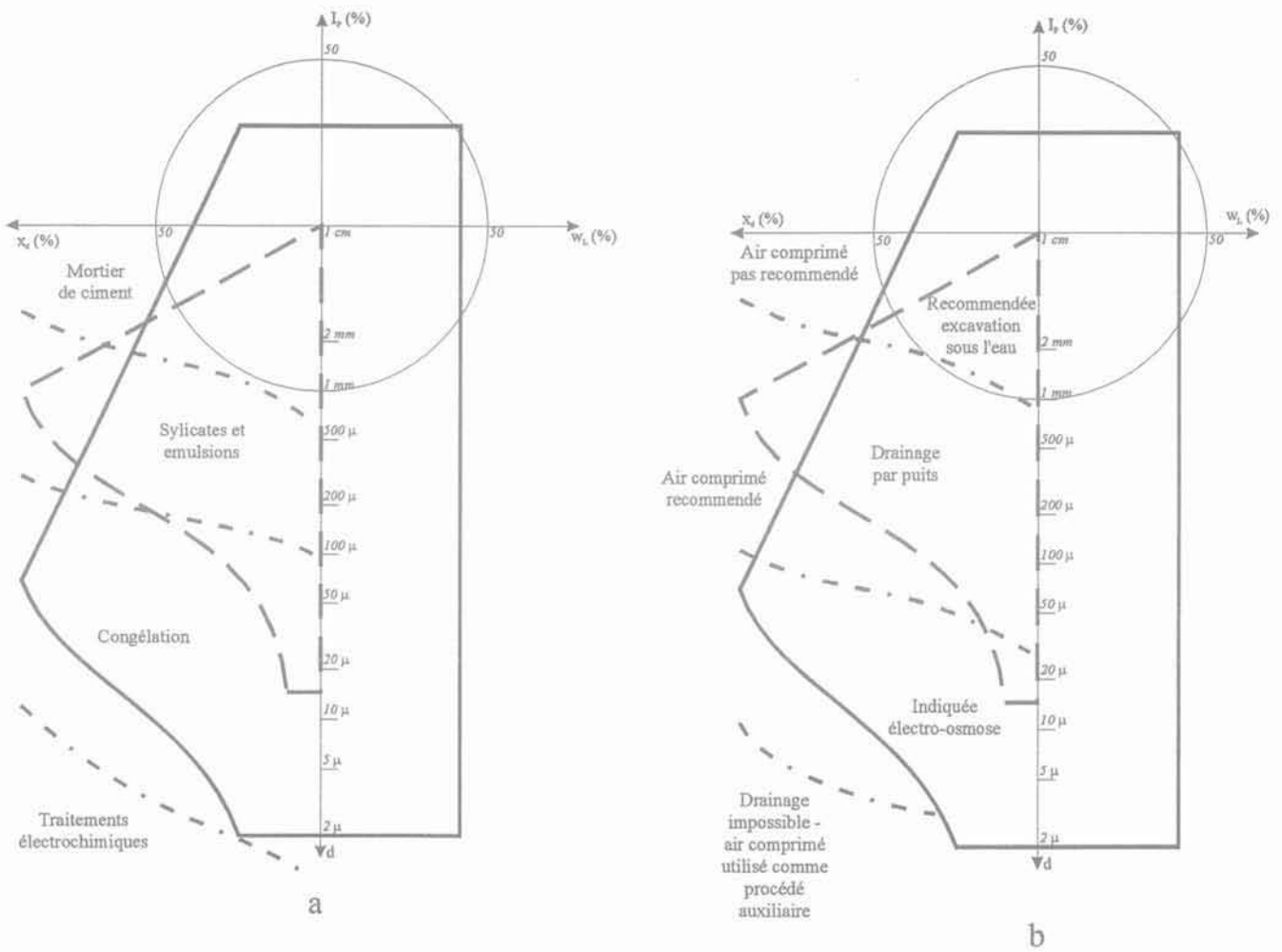
FIG. 5 Les domaines correspondant aux différents procédés de traitement du sol. Domains corresponding to different soil treatment processes.
