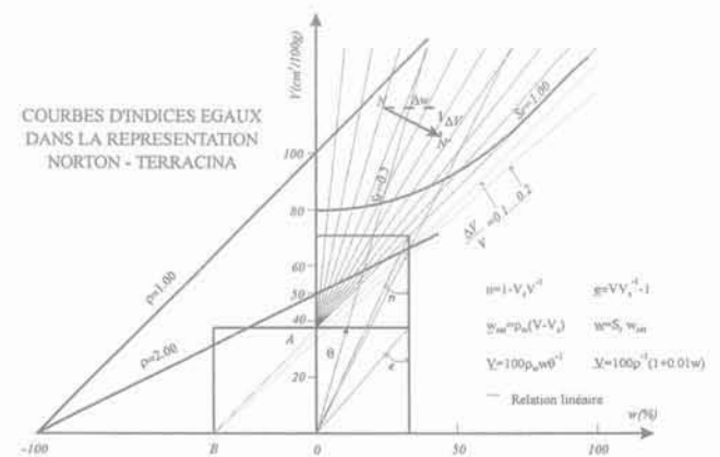
FIG. 7 Le diagramme d'état de Norton-Terracina. Norton-Terracina state diagram.
