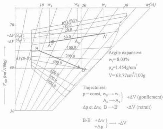
FIG. 14 Diagramme avec les trajectoires d'état d'une argile expansive. Diagram with state paths of an expansive clay.
