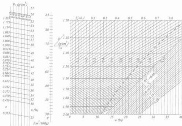
FIG. 8 L'abaque pour le contrôle des résultats des essais. Abacus for the control of test results.
