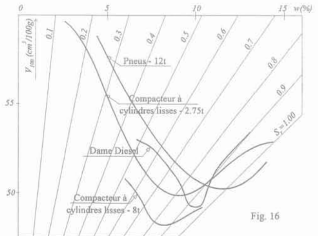
FIG. 16 Diagrammes avec les courbes de compactage d'un tout-venant (a) et d'un sable (b). Diagrams with compaction curves of a gravel-sand-clay mixture (a) and a sand (b).
