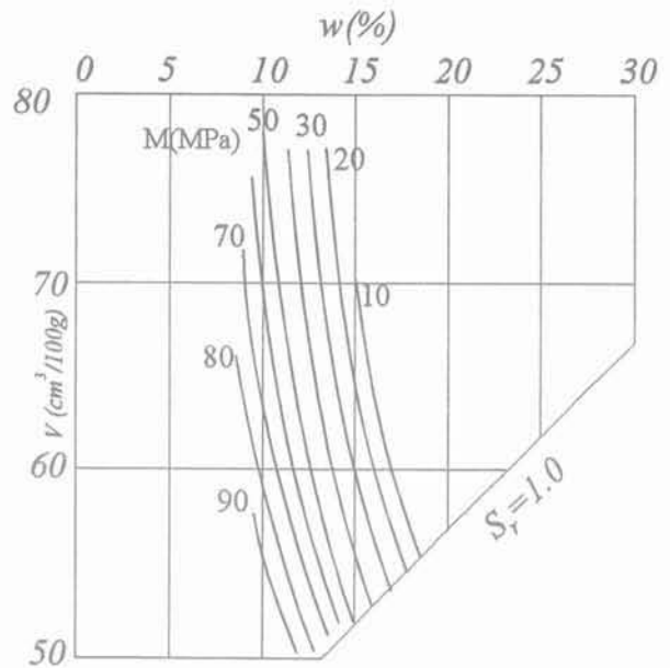
FIG. 9 L'influence de l'état du sol sur le module œdométrique M . Influence of soil state on oedometric modulus M .
