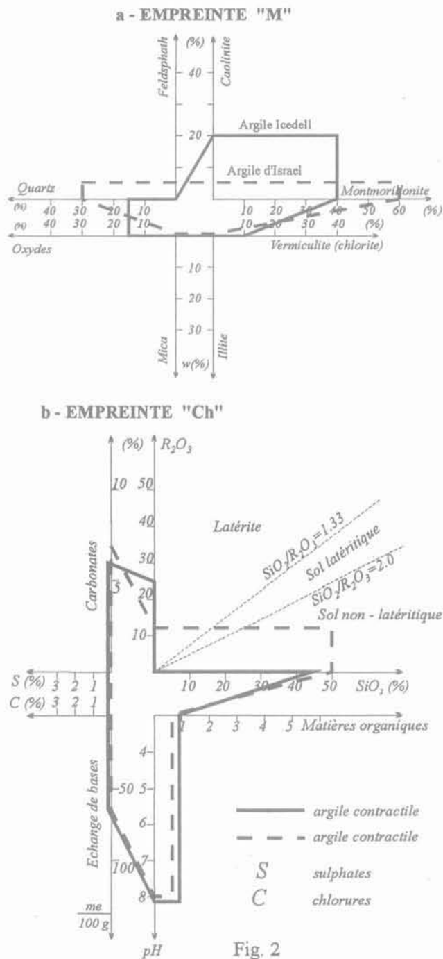
FIG. 2 Les empreintes minéralogiques (« M ») et chimique (« Ch »). Mineralogical (« M ») and chemical (« Ch ») prints.
