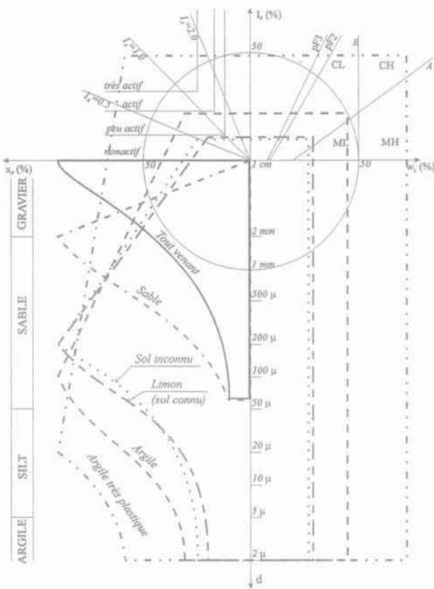
FIG. 15 Empreintes des sols utilisés pour des essais de compactage par le RRL. Prints of soils used in compaction trials by RRL.
