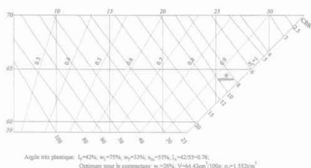
FIG. 20 Diagramme avec courbes d'égal CBR pour une argile très plastique. Diagram with equal CBR curves for a very plastic clay.
