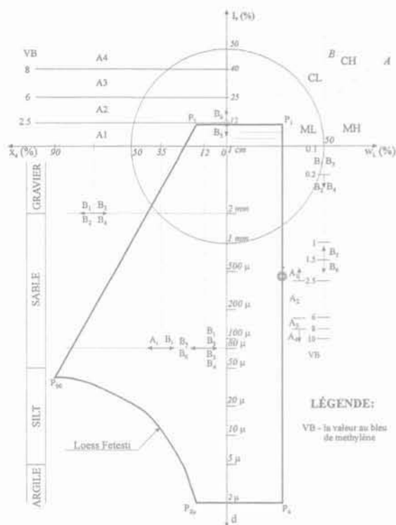
FIG. 3 Les domaines correspondant à la classification française. Domains corresponding to the French classification.
