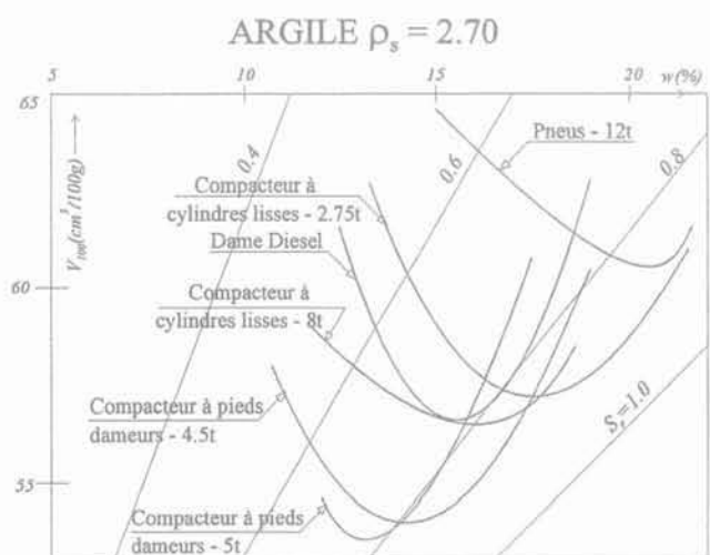
FIG. 17 Diagrammes avec les courbes de compactage d'un silt (a) et d'une argile (b). Diagrams with compaction curves of a silt (a) and a clay (b).
