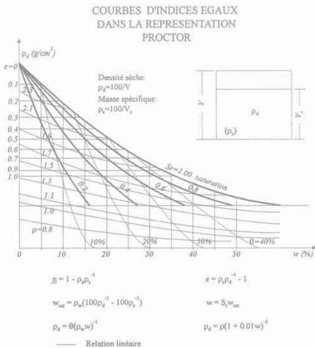
FIG. 6 Le diagramme d'état de Proctor. Proctor's state diagram.
