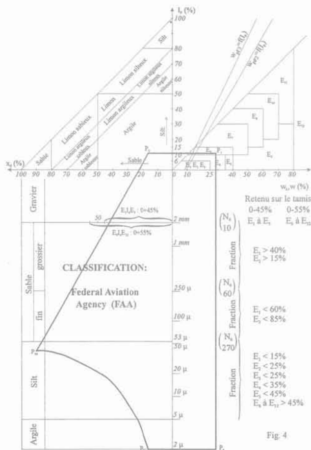
FIG. 4 Les domaines correspondant à la classification américaine FFA. Domains corresponding to the American classification FFA.
