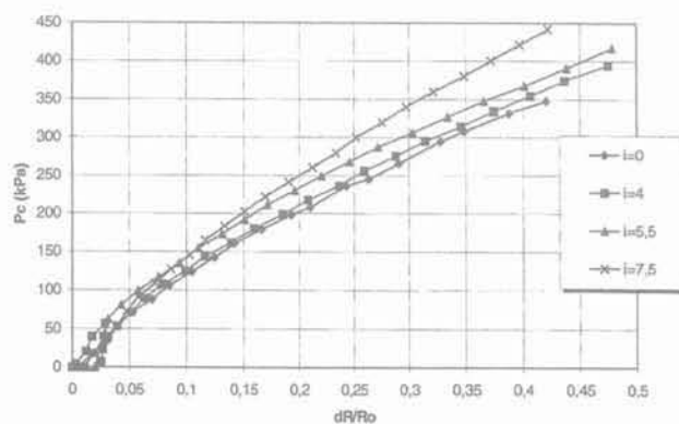
FIG. 3 Courbes d'expansion géomécanométriques ( \gamma = 14,2 \text{ kN/m}^3 , \sigma = 50 \text{ kPa} ). Expansion geomecametric curves ( \gamma = 14.2 \text{ kN/m}^3 , \sigma = 50 \text{ kPa} ).
