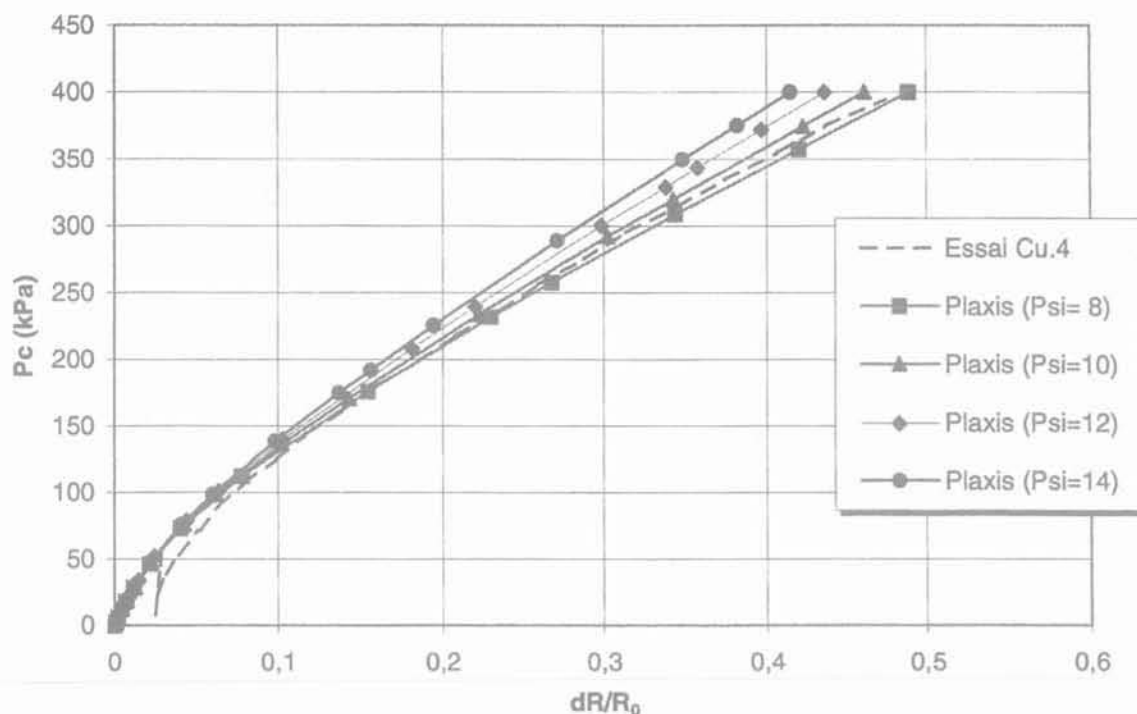
FIG. 13 Influence de l'angle de dilataance \psi pour \phi = 42^\circ . Influence of the dilatancy angle \psi with \phi = 42^\circ .
