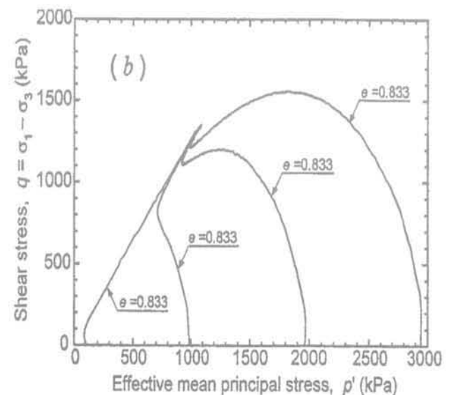
FIG. 6 Influence du niveau de consolidation isotrope sur les comportements observés à l'appareil triaxial (Verdugo, 1992). Influence of the level of isotropic consolidation on the behaviours observed in the triaxial apparatus (Verdugo, 1992).
