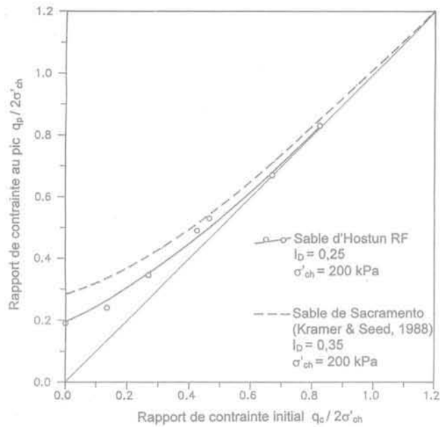
FIG. 7 Influence de l'anisotropie de consolidation sur l'initiation et le développement de la liquéfaction statique (Canou et al. , 1991). Influence of the anisotropy of consolidation on the initiation and development of static liquefaction (Canou et al. , 1991).
