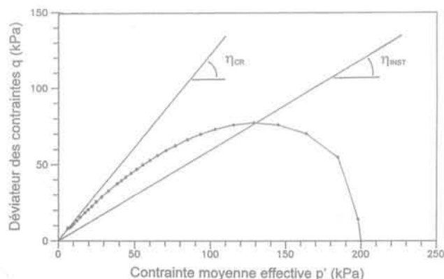
FIG. 4 Essai de liquéfaction statique typique réalisé à l'appareil triaxial (Canou et al. , 1991). Typical static liquefaction test carried out in the triaxial apparatus (Canou et al. , 1991).
