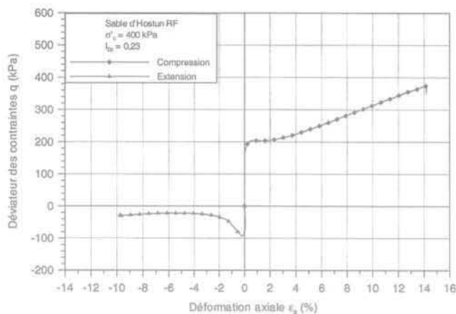
FIG. 8 Influence du trajet de chargement (compression-extension) sur les comportements observés (Benahmed, 2001). Influence of loading path (compression-extension) of the behaviours observed (Benahmed, 2001).
