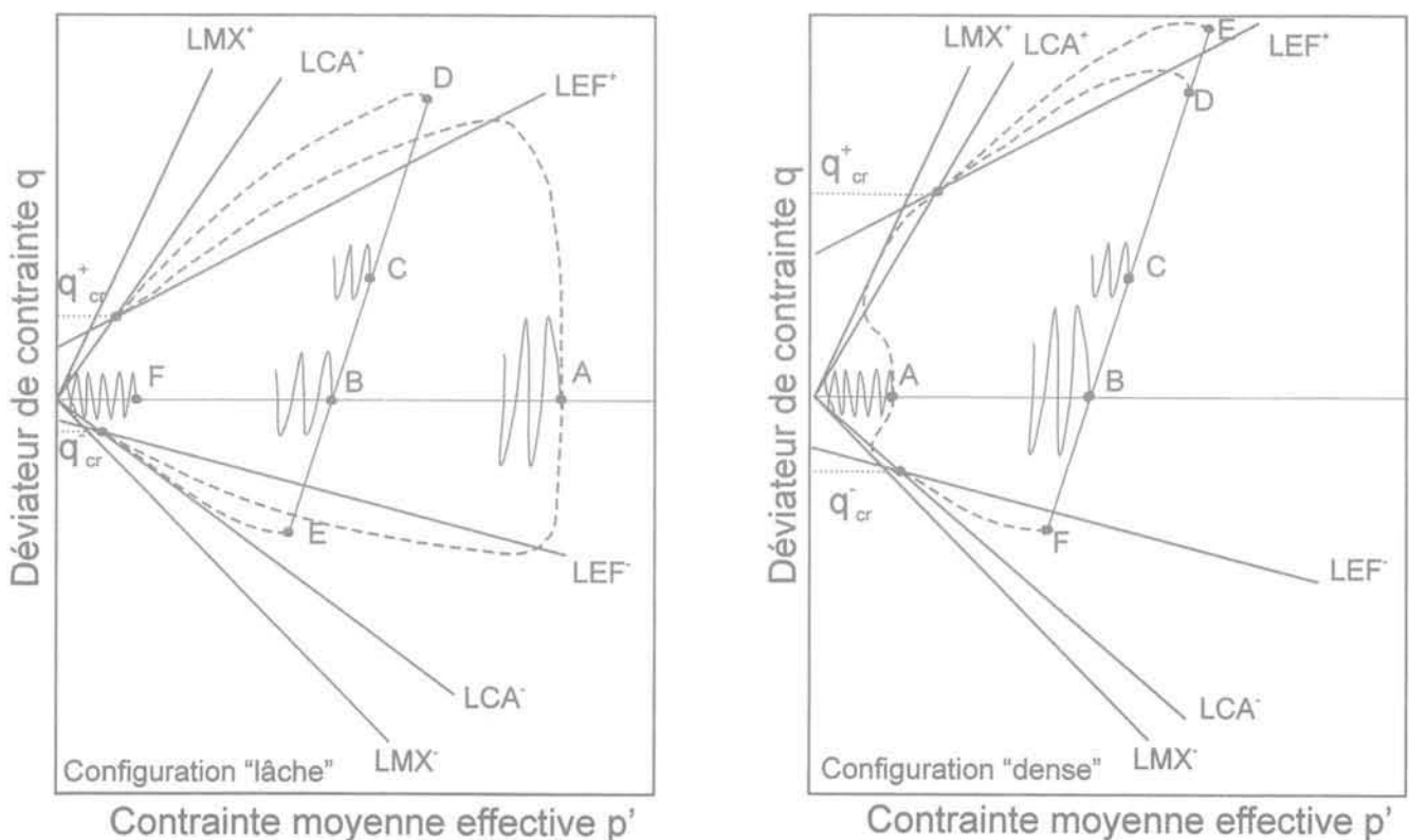
FIG. 17. Cadre conceptuel global (schématique) de prévision du comportement non drainé d'un sable à l'appareil triaxial (configuration « lâche » et « dense »). Global conceptual framework (schematic) for the prediction of the undrained behaviour of a sand, as observed in the triaxial apparatus (« loose » and « dense » configurations).
