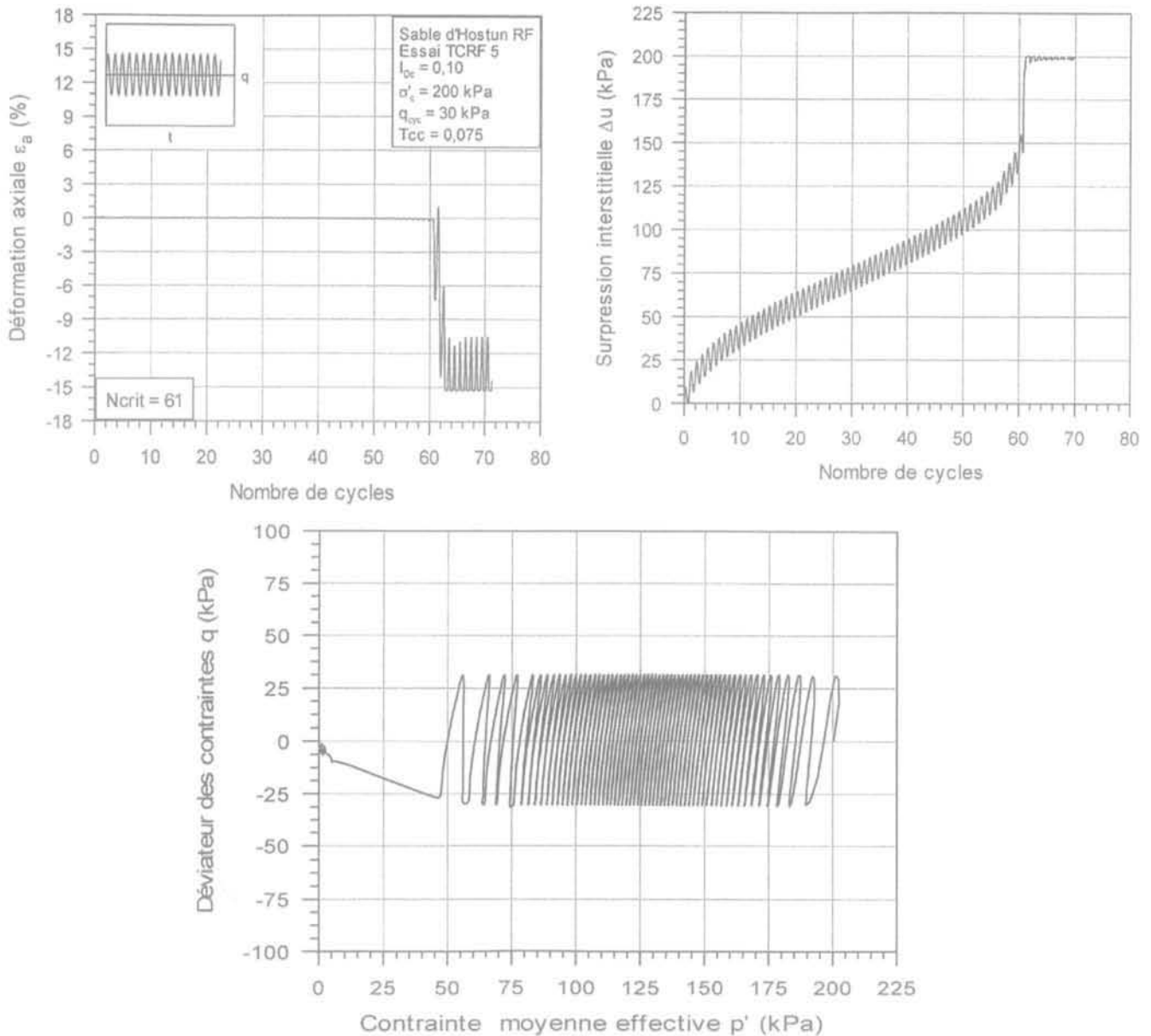
FIG. 16 Comportement typique de liquéfaction cyclique vraie tel qu'observé lors d'un essai triaxial alterné symétrique (Benahmed, 2001). Typical true cyclic liquefaction behaviour as observed in an alternated symmetrical triaxial test (Benahmed, 2001).
