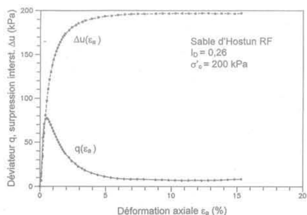
FIG. 4 Essai de liquéfaction statique typique réalisé à l'appareil triaxial (Canou et al. , 1991). Typical static liquefaction test carried out in the triaxial apparatus (Canou et al. , 1991).
