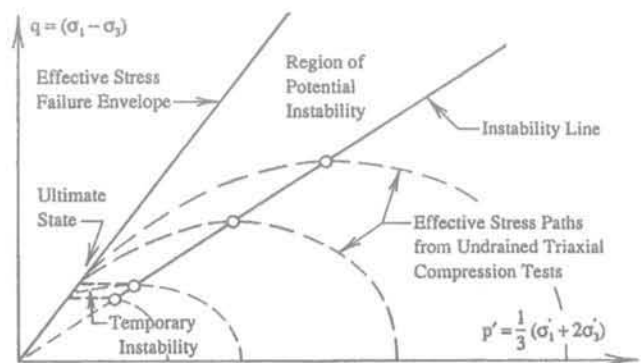
FIG. 11 Ligne d'instabilité de Lade (1992). Instability line, as defined by Lade (1992).
