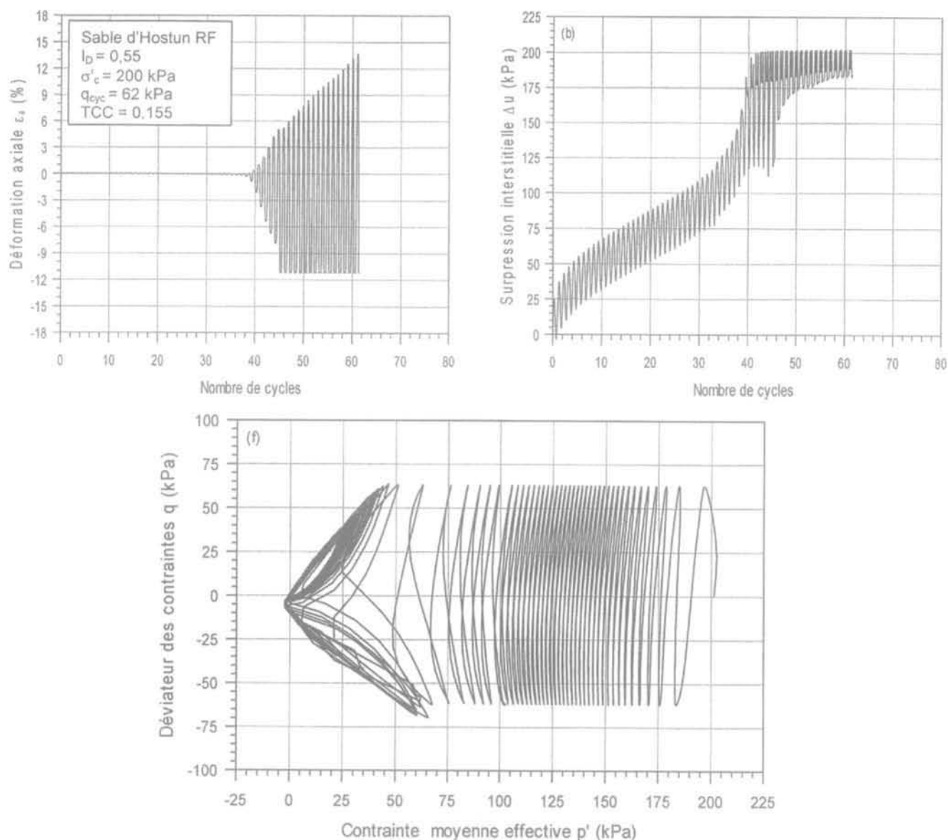
FIG. 15 Comportement typique de mobilité cyclique tel qu'observé lors d'un essai triaxial alterné symétrique (Benahmed, 2001). Typical cyclic mobility behaviour as observed in an alternated symmetrical triaxial test (Benahmed, 2001).
