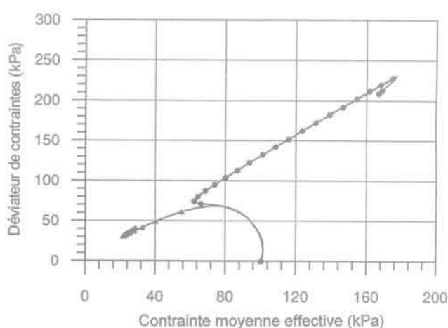
FIG. 9 Influence de la structure sableuse initiale sur les comportements observés (Benahmed, 2001). Influence of initial sand structure on the behaviours observed (Benahmed, 2001).
