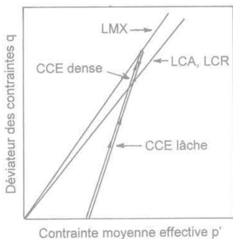
FIG. 2 Comportements typiques observés lors du cisaillement drainé d'un sable en compression à l'appareil triaxial (schématisé). Typical behaviours observed upon drained shear of a sand in compression in the triaxial apparatus (schematic).
