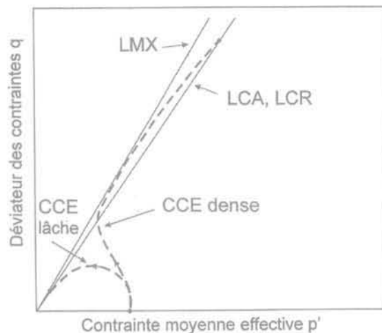
FIG. 3 Comportements typiques observés lors du cisaillement non drainé d'un sable en compression à l'appareil triaxial (schématisé). Typical behaviours observed upon undrained shear of a sand in compression in the triaxial apparatus (schematic).
