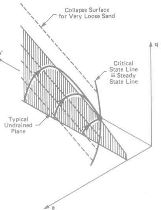
FIG. 10 Définition de la droite et de la surface d'effondrement (Sladen et al. , 1985). Definition of the collapse line and the collapse surface (Sladen et al. , 1985).
