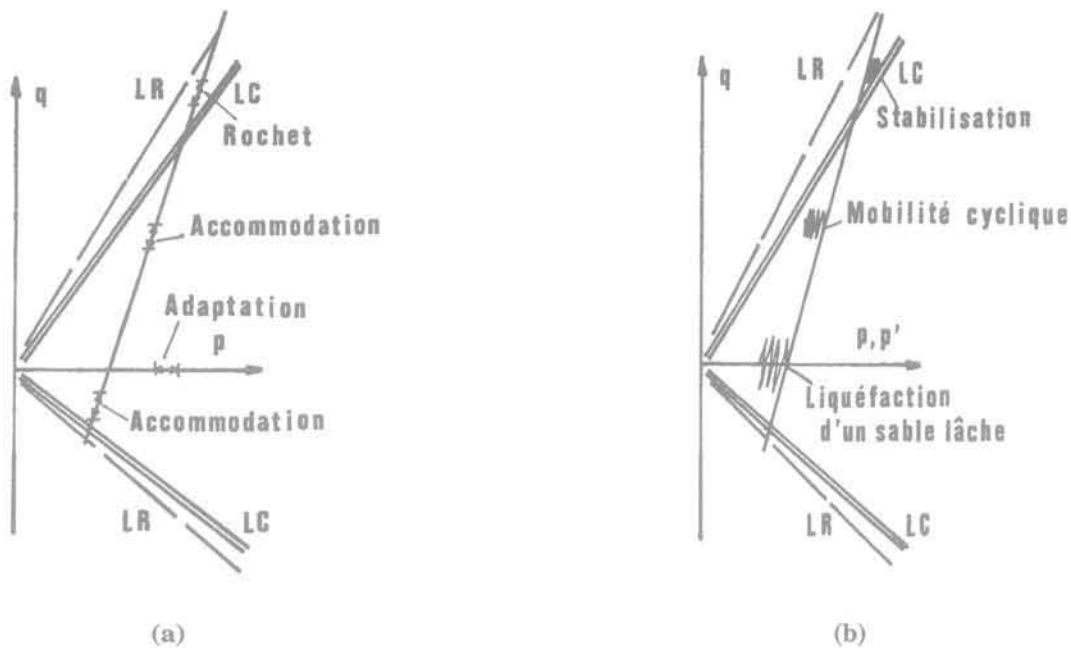
FIG. 14 Cadre conceptuel proposé pour la prévision du comportement cyclique drainé (a) et non drainé (b) des sables (Luong, 1980). Conceptual framework proposed for the prediction of the cyclic behaviour of sands in drained (a) and undrained (b) conditions (Luong, 1980).
