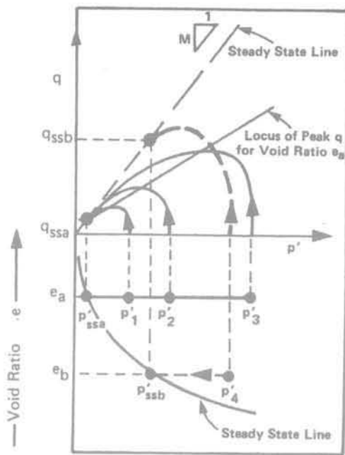
FIG. 10 Définition de la droite et de la surface d'effondrement (Sladen et al. , 1985). Definition of the collapse line and the collapse surface (Sladen et al. , 1985).
