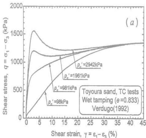
FIG. 6 Influence du niveau de consolidation isotrope sur les comportements observés à l'appareil triaxial (Verdugo, 1992). Influence of the level of isotropic consolidation on the behaviours observed in the triaxial apparatus (Verdugo, 1992).
