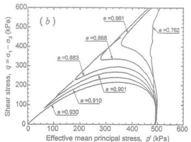
FIG. 5 Influence de l'indice des vides sur les comportements observés à l'appareil triaxial (Verdugo, 1992). Influence of void ratio on the behaviours observed in the triaxial apparatus (Verdugo, 1992).
