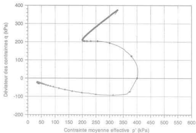
FIG. 8 Influence du trajet de chargement (compression-extension) sur les comportements observés (Benahmed, 2001). Influence of loading path (compression-extension) of the behaviours observed (Benahmed, 2001).
