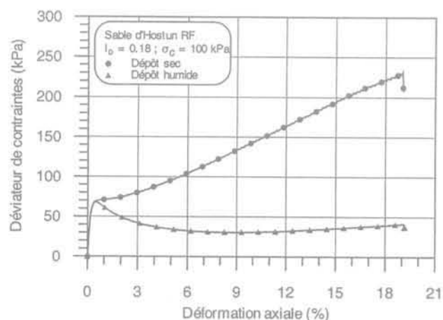
FIG. 9 Influence de la structure sableuse initiale sur les comportements observés (Benahmed, 2001). Influence of initial sand structure on the behaviours observed (Benahmed, 2001).
