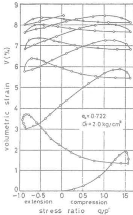
FIG. 13 Mécanismes de densification d'un sable sous cisaillement cyclique à l'appareil triaxial (Tatsuoka et Ishihara, 1974). Densification mechanisms of a sand submitted to a cyclic shear in the triaxial apparatus (Tatsuoka and Ishihara, 1974).
