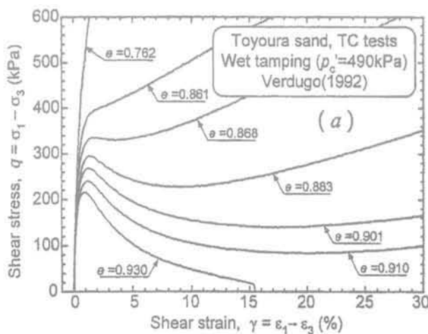
FIG. 5 Influence de l'indice des vides sur les comportements observés à l'appareil triaxial (Verdugo, 1992). Influence of void ratio on the behaviours observed in the triaxial apparatus (Verdugo, 1992).
