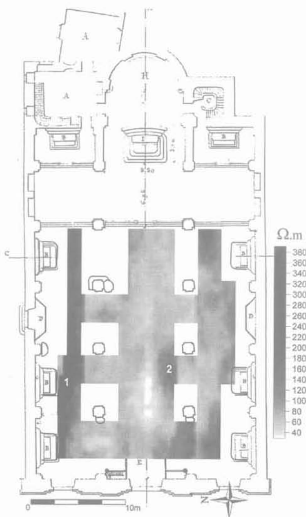
FIG. 5. Prospection électrostatique avec le petit quadripôle ( a = 0,60 m) dans la cathédrale Sainte-Marie de Bastia. Electrostatic survey with small four poles array ( a = 0,60 m) in Sainte-Marie cathedral at Bastia.
