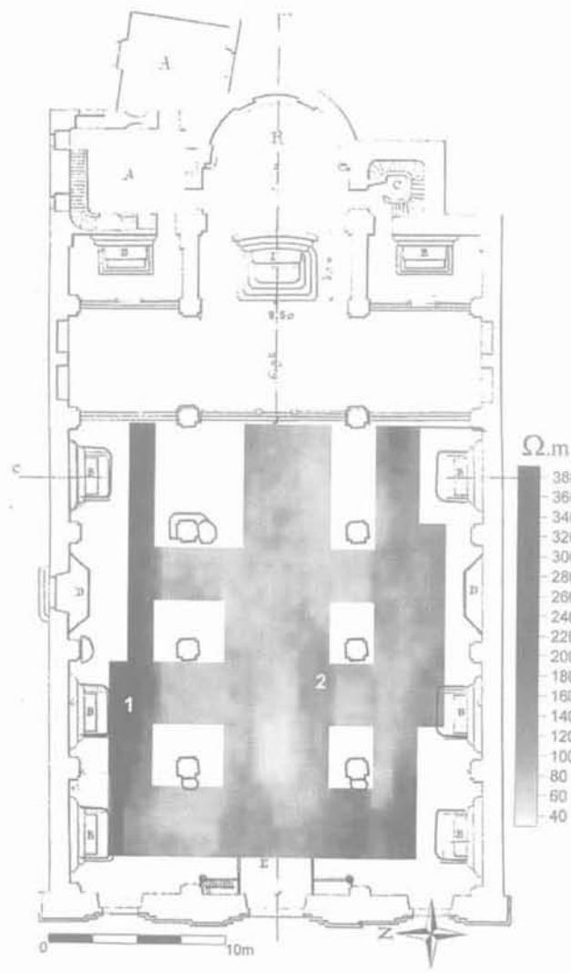
FIG. 6. Prospection électrostatique avec le grand quadripôle ( a = 1,50 m) dans la cathédrale Sainte-Marie de Bastia. Electrostatic survey with main four poles array ( a = 1,50 m) in Sainte Marie cathedral at Bastia.
