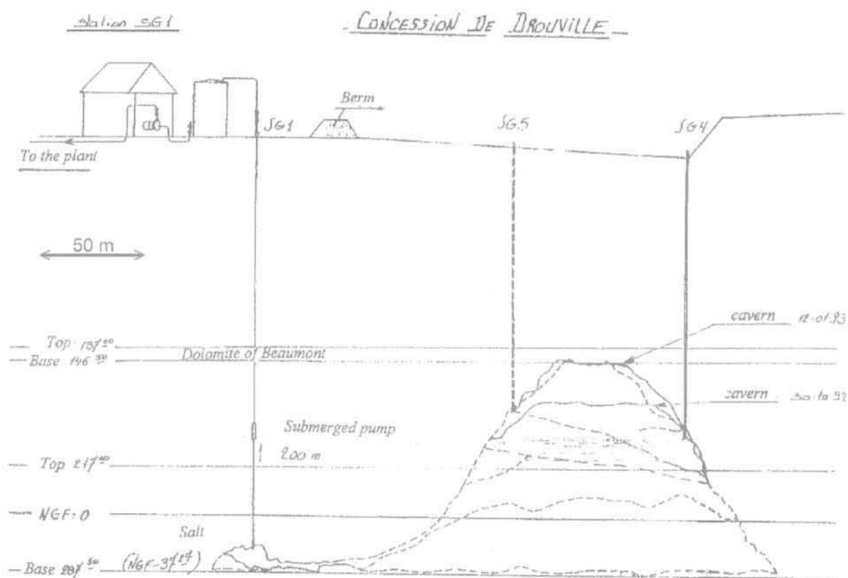
FIG. 7 Pompage de la saumure dans les cavernes SG4-SG5 (concession de Drouville). Le toit de la caverne remonte jusqu'à la Dolomite de Beaumont, atteinte en 1992. On décide alors de décompresser la caverne en descendant le niveau de saumure dans le puits SG1 au moyen d'une pompe immergée. La chute de pression dans la caverne n'a pas provoqué l'effondrement (d'après Buffet, 1998). Brine withdrawal from the SG4-SG5 caverns (Drouville concession). Cavern roof rises through stoping and reaches the Beaumont Dolomite by 1992. It was decided to lower brine level in SG1 well. A submerged pump was used. Pressure drop did not provoke cavern failure (After Buffet, 1998).
