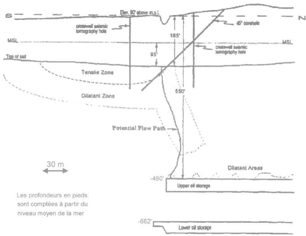
FIG. 3 Mine de sel de Weeks Island, convertie en stockage de pétrole. La modélisation géomécanique de Ehgartner et Hoffman montre le mécanisme de développement d'une fissure en traction au-dessus des vides miniers après plusieurs années, et sa progression à travers les zones dilatantes endommagées (d'après Bauer et al. , 2000).
