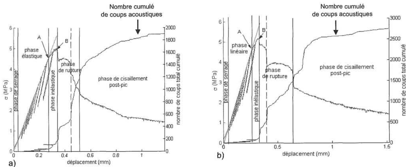
FIG. 5 Évolution du nombre de coups cumulés d'émission acoustique au cours de la déformation de deux essais de craies.
