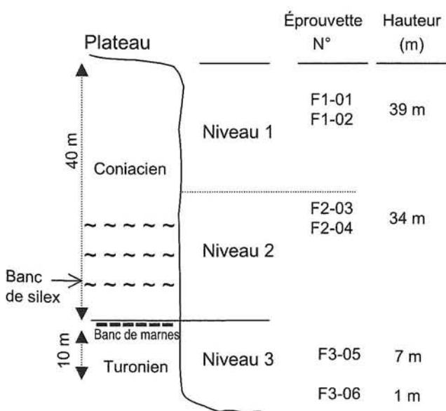
FIG. 1 Série lithologique simplifiée du front de la falaise avec la localisation des échantillons prélevés aux différents niveaux de la falaise.
