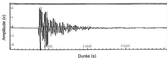
FIG. 4 Exemple d'une trace sismique enregistrée lors d'un essai.
