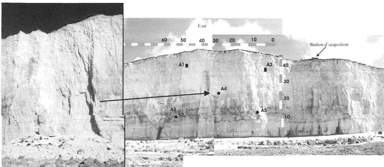
FIG. 7 Localisation du réseau de capteurs microsismiques installés au front de la falaise et illustration de l'éboulement apparu au centre de la zone instrumentée.
