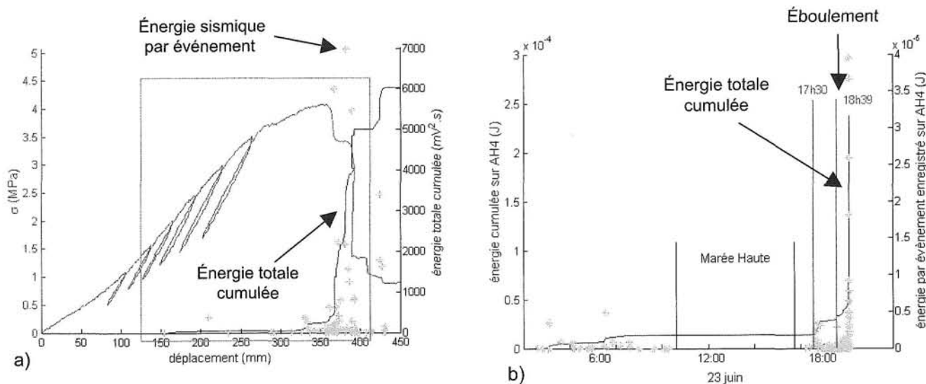
FIG. 8 Évolution de l'énergie sismique cumulée : (a) en laboratoire, (b) sur le site de Mesnil-Val.
