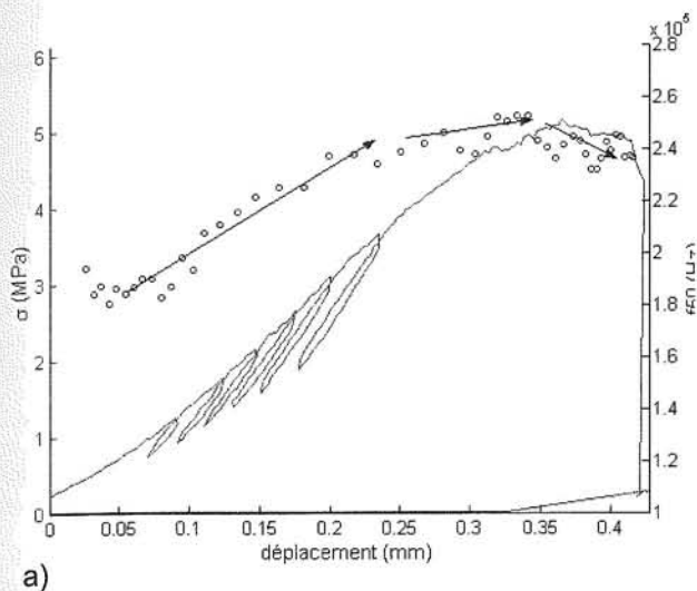
FIG. 9 Évolution de la fréquence centrale des signaux enregistrés : (a) en laboratoire (b) sur le site avant et pendant l'éboulement.
