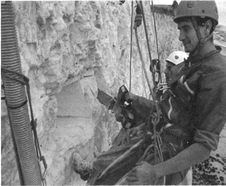
FIG. 2 Prélèvement des blocs de craie au front de la falaise de Mesnil-Val.
