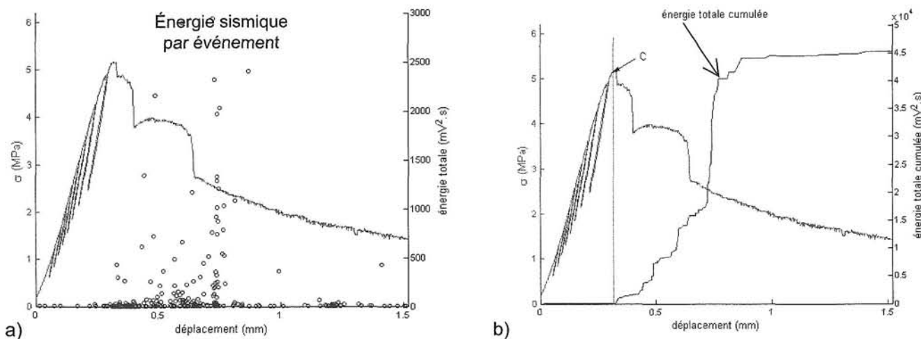
FIG. 6 Corrélation entre l'énergie par événement (a), l'énergie cumulée (b) et la déformation de l'éprouvette.
