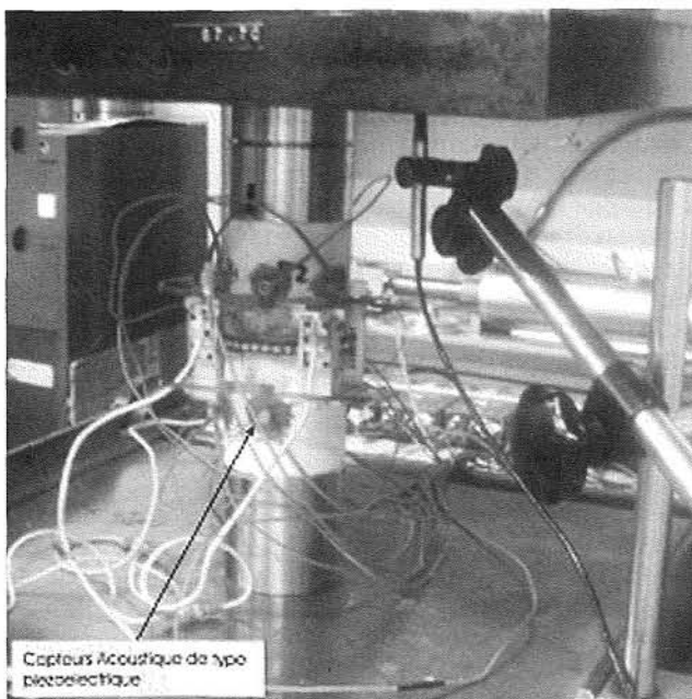
FIG. 3 Configuration des capteurs acoustiques autour de l'échantillon.
