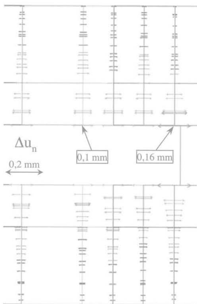
FIG. 5 Fermetures mécaniques et déplacements tangentiels des fractures induits par le creusement de la galerie dans le cas du modèle de référence. Fracture mechanical closures and fracture shear displacements induced by the excavation of the storage gallery (reference case).
