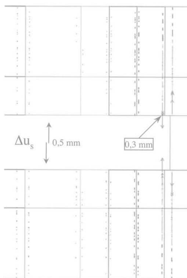
FIG. 5 Fermetures mécaniques et déplacements tangentiels des fractures induits par le creusement de la galerie dans le cas du modèle de référence. Fracture mechanical closures and fracture shear displacements induced by the excavation of the storage gallery (reference case).
