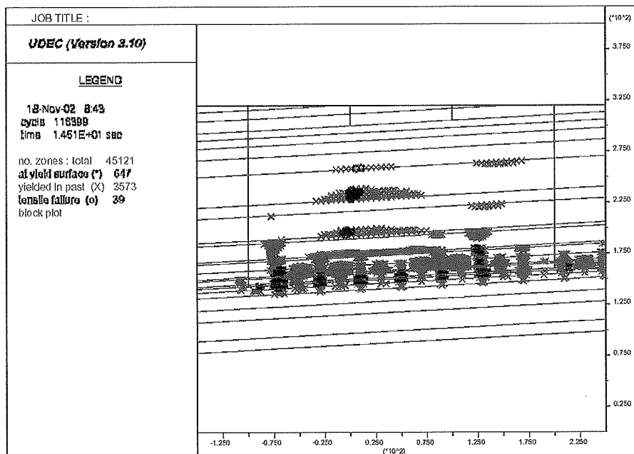
FIG. 11 Développement des points en rupture suite au dégraissage des piliers (phase 3). Failure points development due to re-mining of pillars (phase 3).
