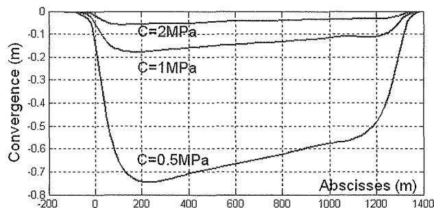
FIG. 14 Convergence calculée dans les chantiers peu profonds en fonction de la valeur attribuée à la cohésion du charbon.
