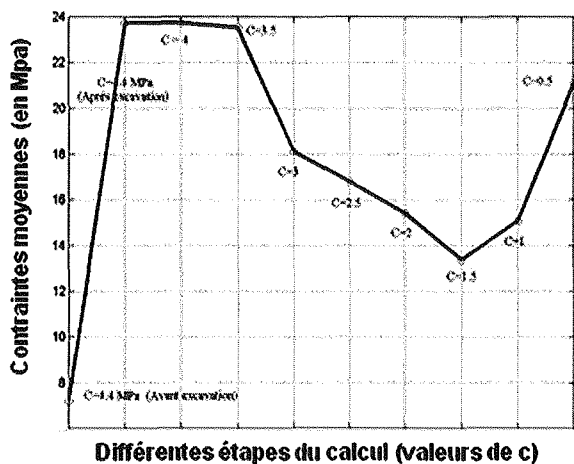
FIG. 13 Évolution de la contrainte moyenne au sommet d'un pilier situé au centre d'un panneau profond situé avant exploitation (cas 1) et, après exploitation, pour des valeurs de cohésion de charbon variant de 4 à 0,5 MPa (autres cas).
