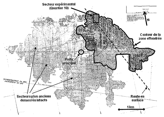
FIG. 3 Plan de la mine au moment de l'effondrement. Les zones en gris plus foncé ont été reprises sur le même principe que l'expérimentation menée au sein de « quartier 10 » (d'après Van der Merwe, 2006b). Map of the mine at the time of the collapse. The darker grey sectors have been re-mined on the same principle of what has been performed in experimental « sector 10 » (from Van der Merwe, 2006b).
