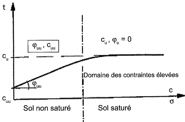
FIG. 2.3 Critère de rupture en conditions non drainées (Philipponnat, 2006).
