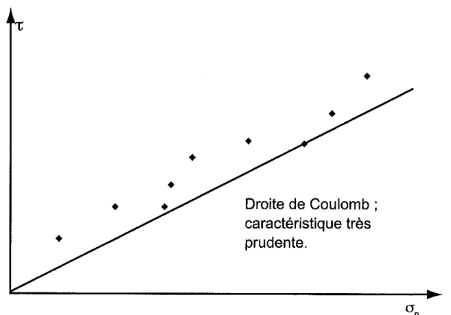
FIG. 2.8 Interprétation d'une série d'essais triaxiaux réalisés sur un sol de fondation hétérogène.
