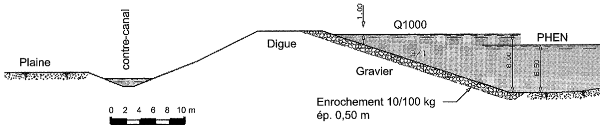
FIG. 5.2 Coupe type d'une digue (solicitations hydrauliques normales).
