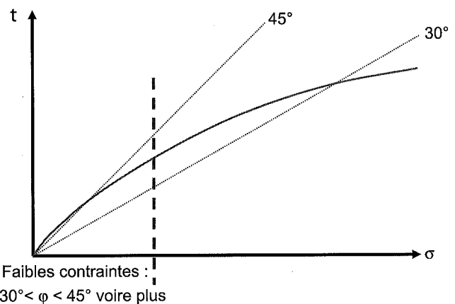
FIG. 2.5 Courbe intrinsèque parabolique pour un enrochement.
