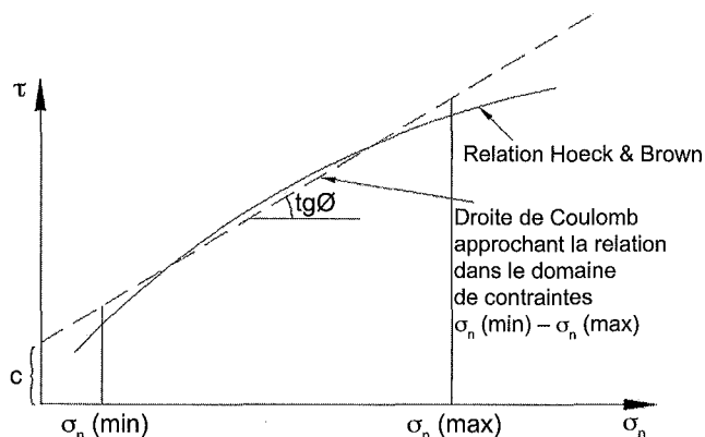
FIG. 2.6 Droite de Coulomb approchant la relation de Hoek et Brown pour déterminer c_{\text{fond}} et \varphi_{\text{fond}} .
