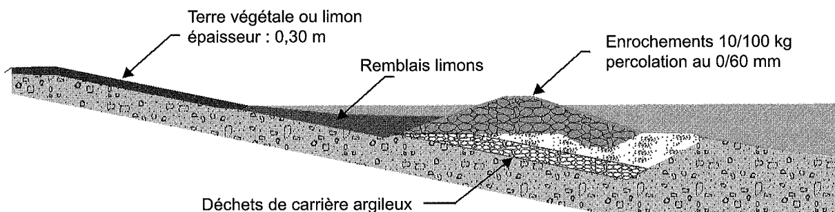
FIG. 5.4 Exemple de protection de talus avec végétation.
