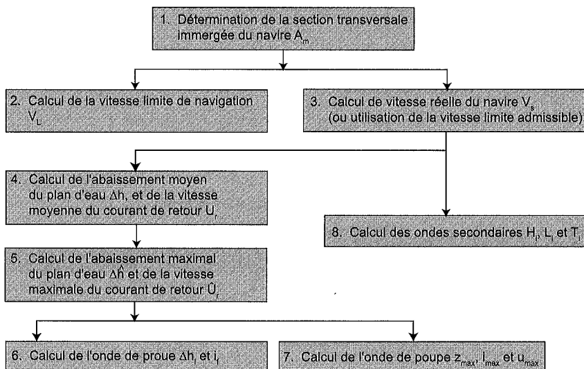
FIG. A.4.4 Diagramme de calcul des mouvements de l'eau induits par la navigation (guide Enrochements , 2009).
