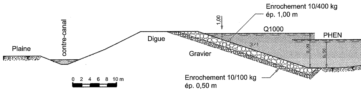
FIG. 5.3 Coupe type d'une digue (solicitations hydrauliques fortes).
