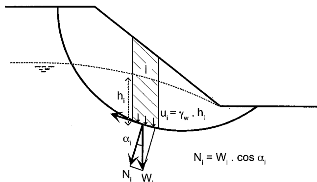
FIG. 4.1 Principe de calcul de la stabilité dans le cas d'une surface de rupture circulaire.
