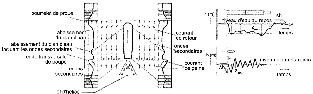
FIG. A.4.3 Caractéristiques des mouvements induits par la navigation par rapport à la stabilité des berges (guide Enrochements , 2009).
