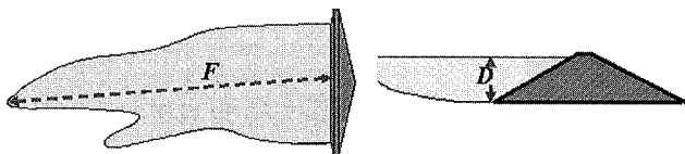
FIG. A.4.2 Fetch et profondeur du plan d'eau.
