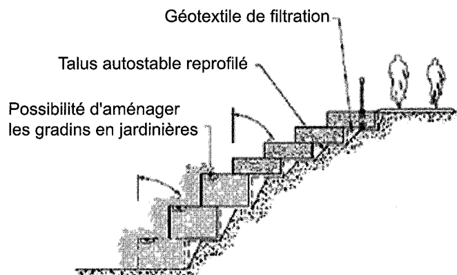
FIG. A.7.1 Exemple de protection de berges : a) matelas Réno ; b) gabions végétalisés.
