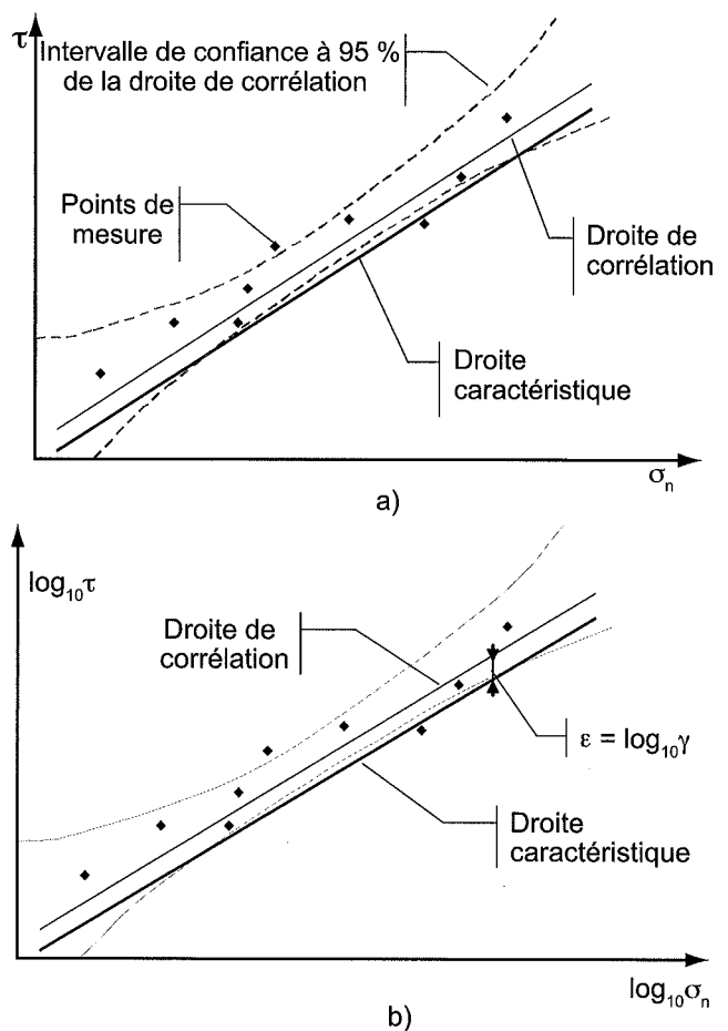
FIG. 2.7 Interprétation d'une série d'essais triaxiaux réalisés sur un sol de remblai homogène, (a) en échelle arithmétique et (b) en échelle logarithmique.
