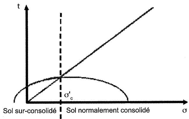
FIG. 2.4 Courbe intrinsèque pour un sol fin.
