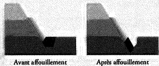
FIG. A.5.1 Protection d'une digue au moyen d'une carapace et d'une banquette (appelée aussi sabot ou bêche parafouille) en enrochements (source CETE Méditerranée).
