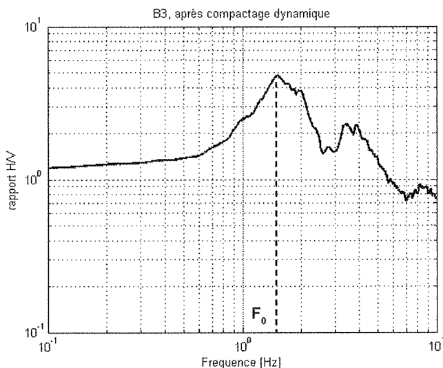
FIG. 4 Détermination de F_0 après rapport des deux composantes horizontales sur la composante verticale des amplitudes spectrales du bruit sismique enregistré.
