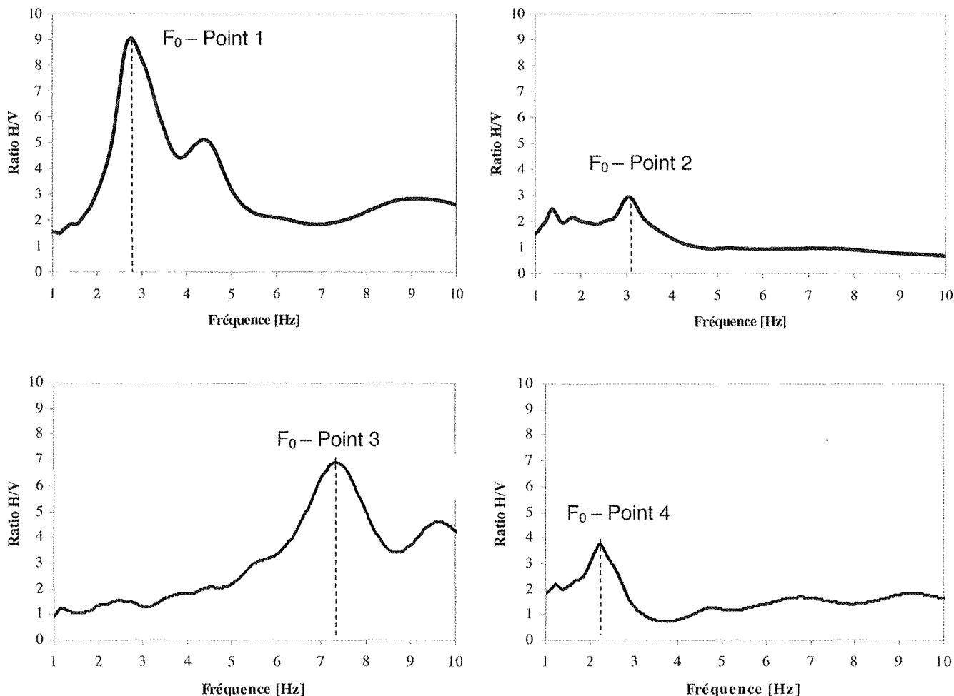
FIG. 9 Détermination de F_0 à partir des rapports spectraux H/V issus de mesures de bruit de fond sismique dans la Vallée du Rhône. Identification of F_0 using H/V ratio based on seismic noise records in Rhône Valley.
