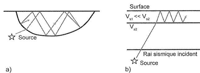
FIG. 2 Schéma de principe du piégeage des ondes avec analogie optique du rai incident et réfléchi. a) Piégeage à l'échelle d'un bassin sédimentaire. b) Piégeage dans une formation superficielle, avec V_{s1} et V_{s2} les vitesses des ondes de cisaillement dans les formations 1 et 2.
