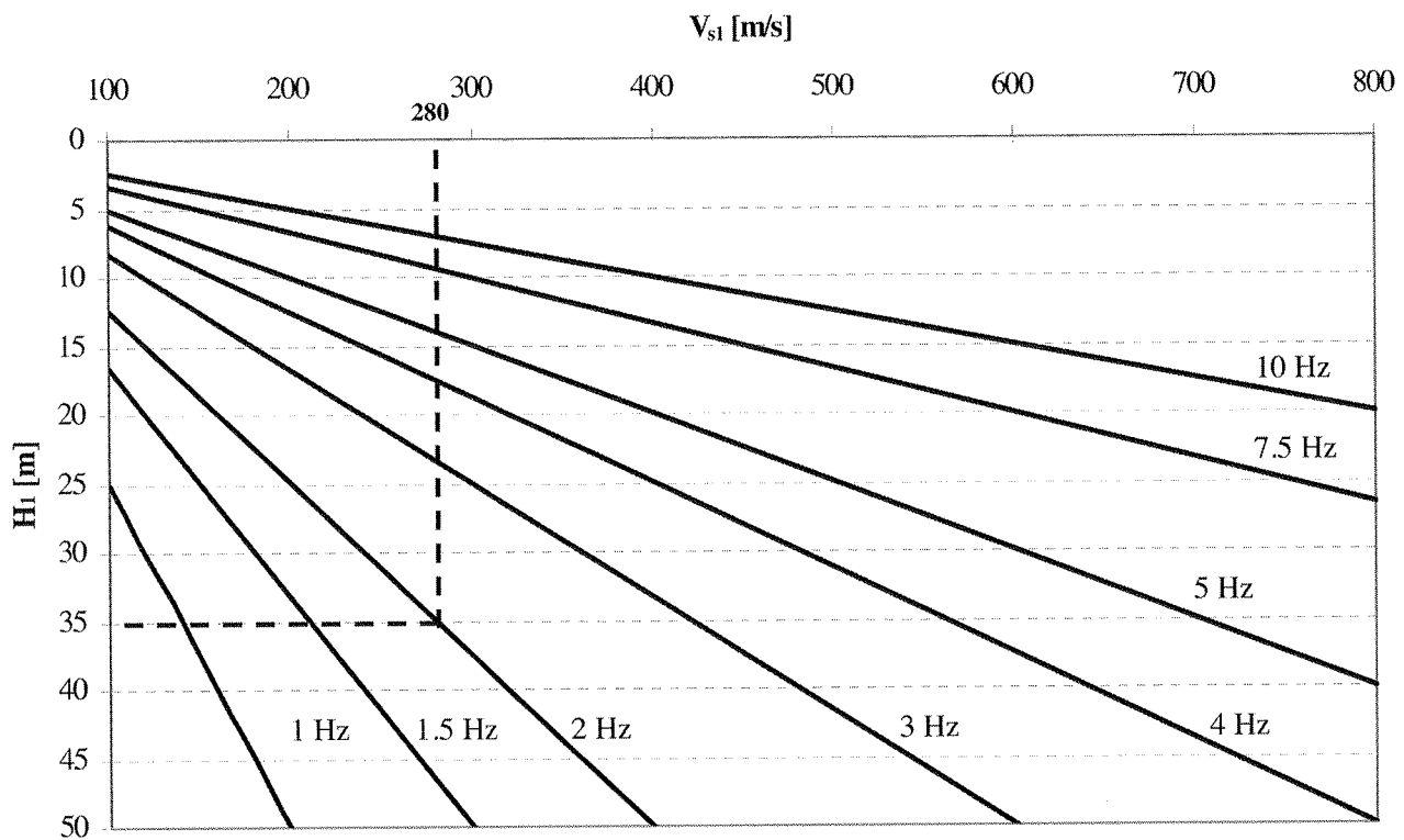
FIG. 6 Abaque ( H_v, V_{s1}, F_0 ) pour un modèle de sol bicouche tel que \rho_2 \cdot V_{s2} / \rho_1 \cdot V_{s1} > 4 . Abacus ( H_v, V_{s1}, F_0 ) for a two layers model in case of \rho_2 \cdot V_{s2} / \rho_1 \cdot V_{s1} > 4 .
