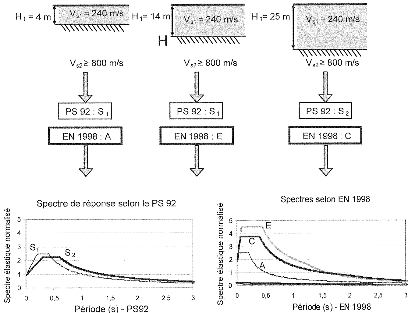
FIG. 3 Effet de la variation d'épaisseur d'une couche superficielle ( V_{s1} de 240 m/s) surmontant un substratum rocheux ( V_{s2} > 800 m/s) sur la classe de sol et le spectre de réponse normé calculé avec un amortissement de 5 %, selon deux règlements (Règles PS92 et EN 1998). EN 1998, cas d'un bâtiment de catégorie d'importance II. PS92, cas d'un bâtiment de classe B.
