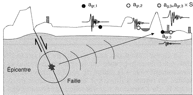
FIG. 1 Schéma de principe décrivant la rupture d'une faille qui engendre des ondes sismiques dont l'amplitude varie en particulier avec la distance épacentrale ( a_{gr,3} < a_{gr,2} < a_{gr,1} ) et selon les conditions géologiques locales ( a_{g,3} > a_{gr,3} ). S représente l'augmentation de l'accélération due à l'effet de site.
