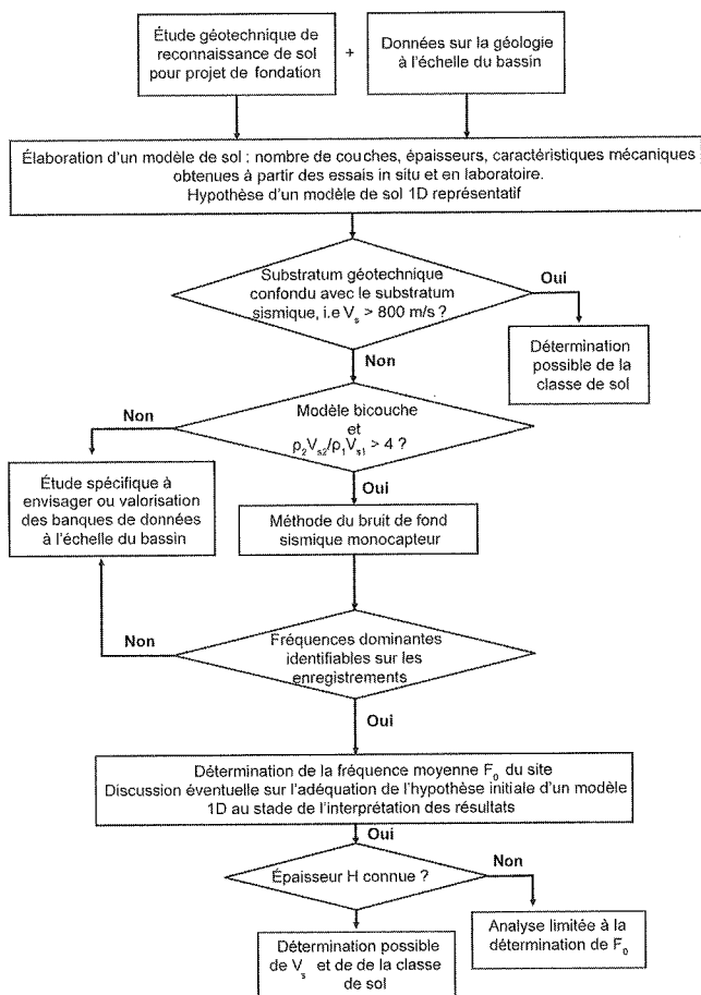
FIG. 7 Principe de l'utilisation conjointe de la mesure du bruit de fond à l'étude géotechnique pour un modèle de sol bicouche.
