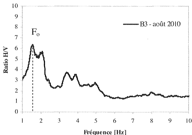
FIG. 11 Détermination de F_0 à partir des mesures de bruit de fond sismique dans la vallée du Gier. Identification of F_0 using seismic noise records in Gier Valley.
