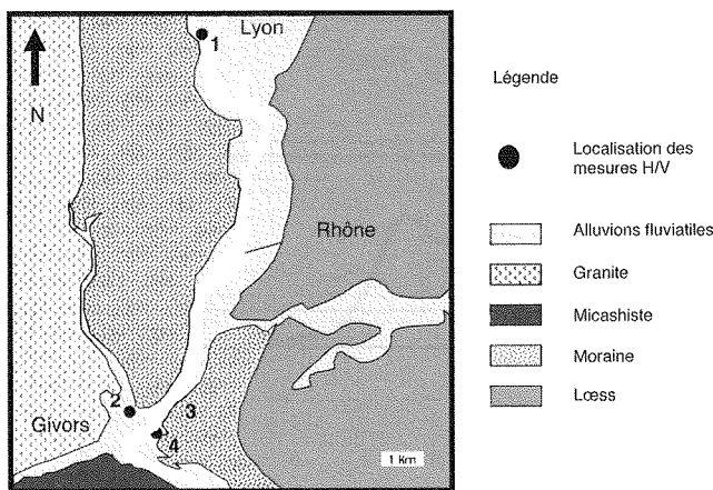
FIG. 8 Carte géologique simplifiée de la vallée du Rhône au sud de Lyon et emplacements des mesures du bruit de fond sismique. Simplified geological map of the Rhône river valley south of Lyon City and location of seismic noise measurements.
