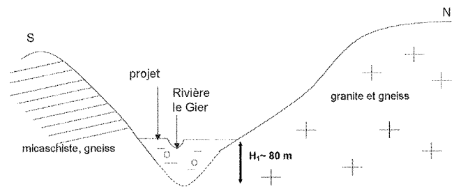
FIG. 10 Géomorphologie de la vallée du Gier vers la confluence avec le Rhône.
