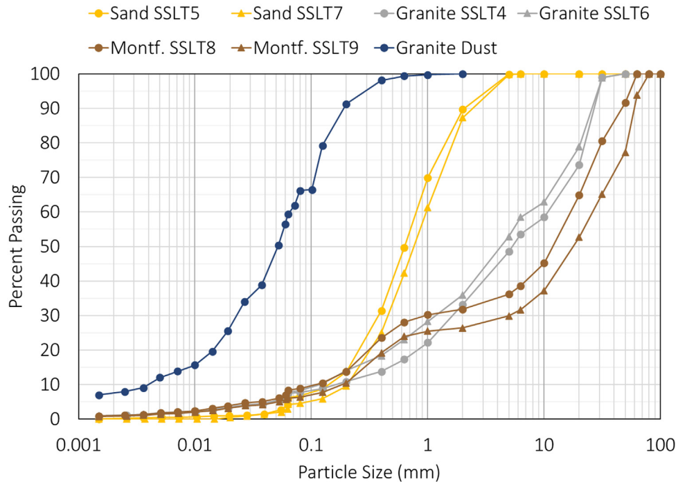
Fig. 2. Granulométrie des matériaux utilisés pour construire les remblais à petite échelle. Fig. 2. Grain size of materials used to build small-scale embankments.
