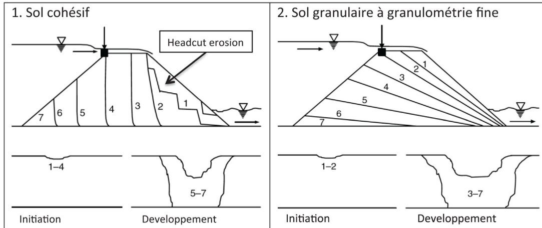
Fig. 1. Illustration des mécanismes d'érosion par surverse par « Headcut Migration » (à gauche) et par érosion de surface (à droite). Fig. 1. Illustration of headcut migration (left) and surface erosion (right) mechanisms.
