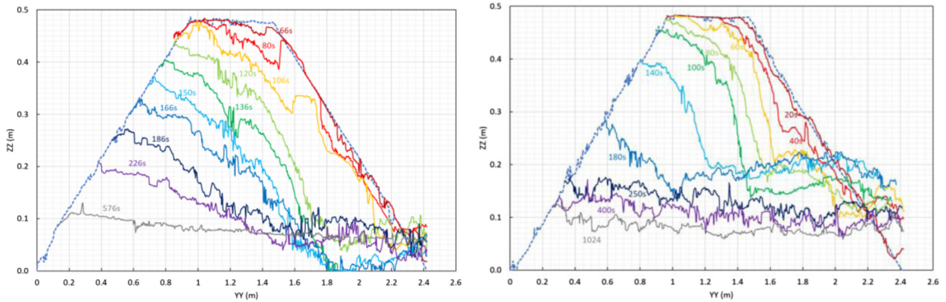
Fig. 3. Profils d'érosion du remblai en sable (gauche) et du remblai en graviers de granite (droite). Fig. 3. Erosion profiles of sand fill (left) and granite gravel fill (right).
